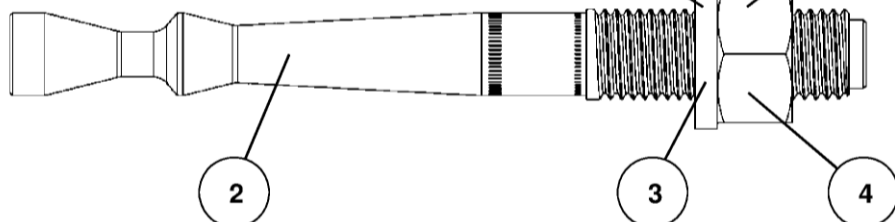
fischer Highbond- Ankerstange FHB II Inj-A S Größe: M10, M12, M16, M20, M24
