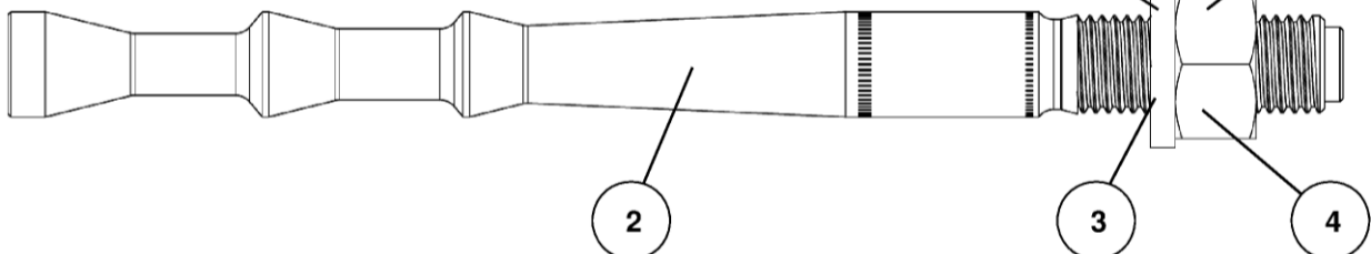
fischer Highbond- Ankerstange FHB II Inj-A L Größe: M8, M10, M12, M16, M20, M24
