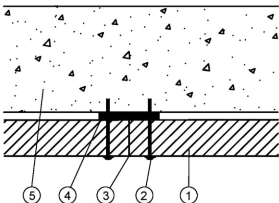
Schnitt Decke mit Bekleidung aus Brandschutzplatten
