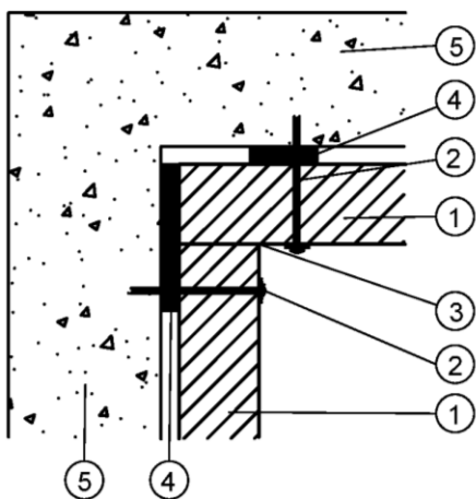
Detail Befestigung Bekleidung aus Brandschutzplatten
