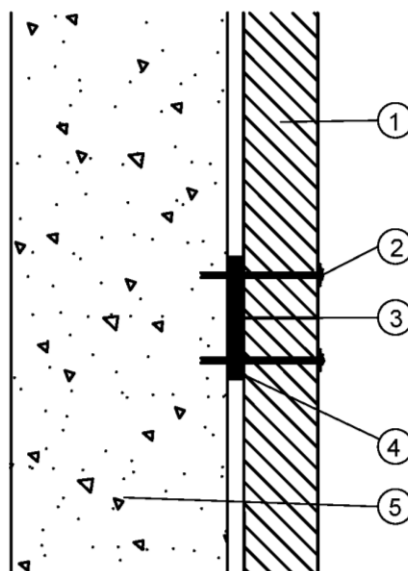
Schnitt Wand mit Bekleidung aus Brandschutzplatten
