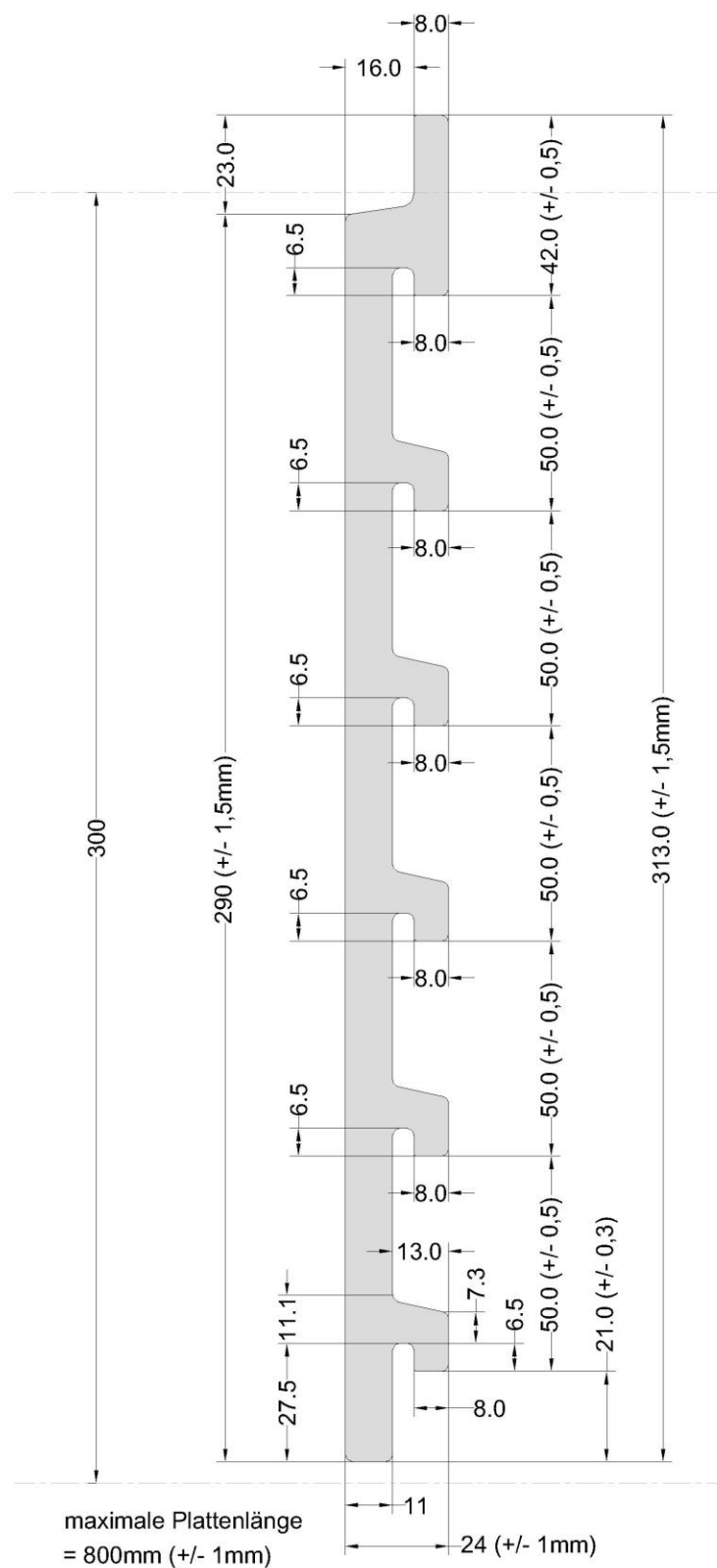
Vorgehängtes hinterlüftetes Fassadensystem "Argelite"
