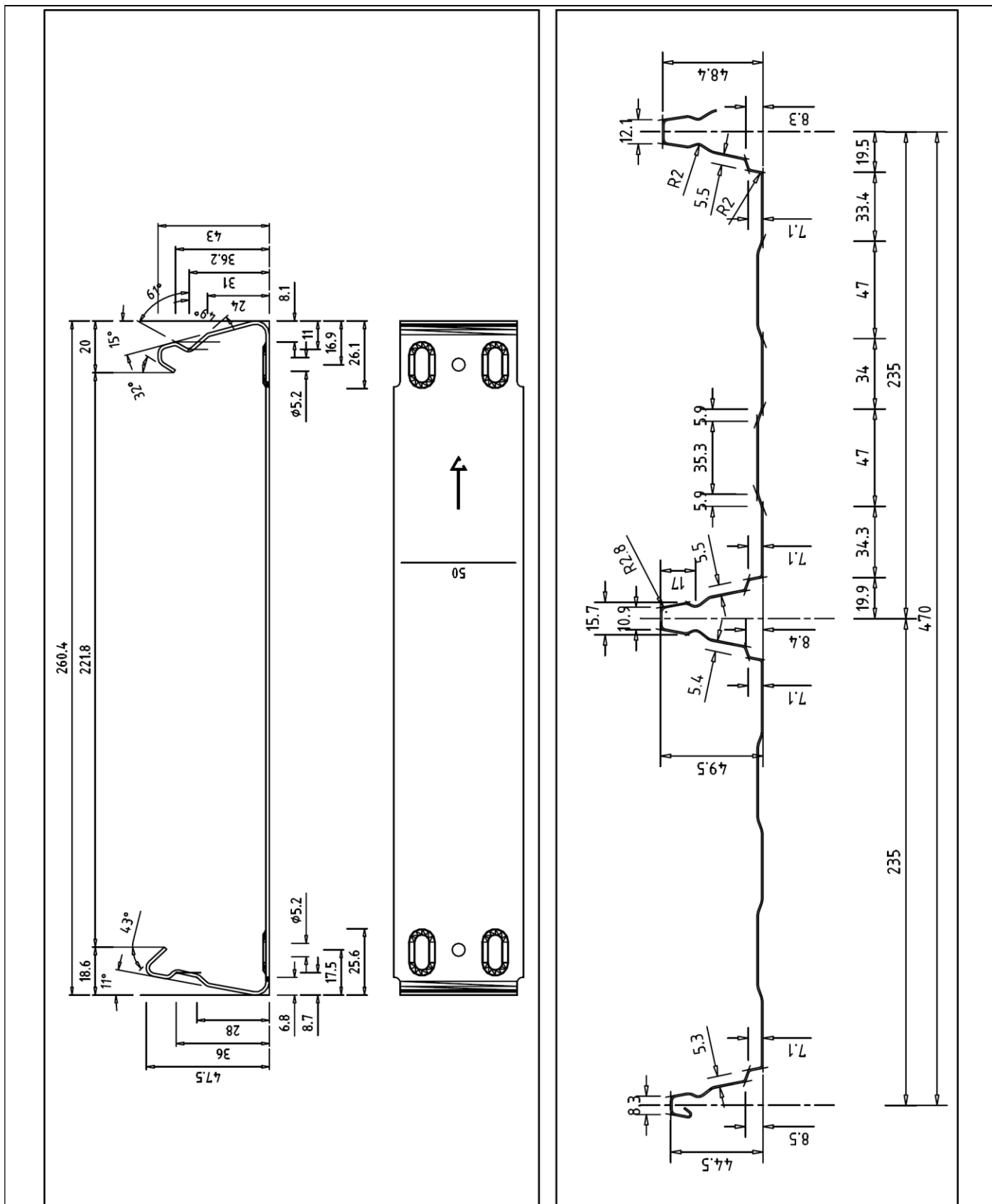
GBS-Klemmrippenprofil-Dachelemente aus Aluminium
