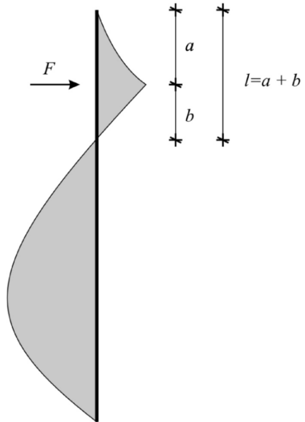
Momentenverlauf
