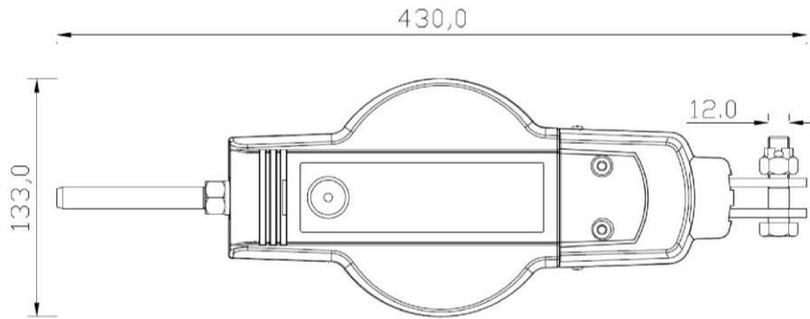
85700-00 18 kN Falldämpfer zum Verpressen
