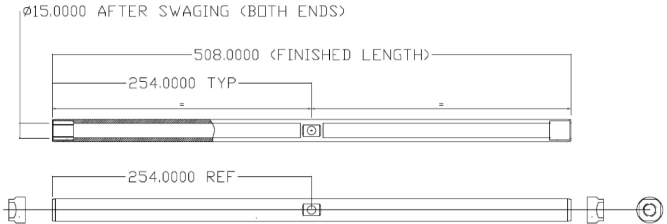
85651-00 Spannhülse, verlängert
