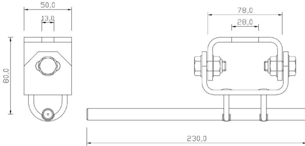
85062-00 Seilhalter für Eckumfahrungen, einseitig verlängertes Röhrrchen (M12 Verschraubung)
