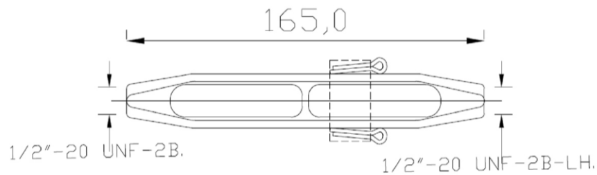
85050-00 Spannhülse
