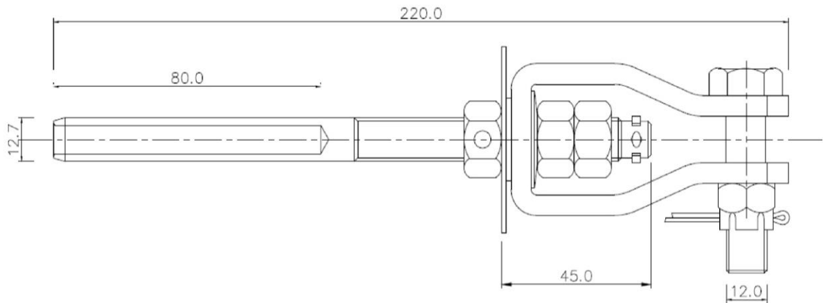
85390-00 Anzeigenscheibe für die Seilvorspannung zum Verpressen
