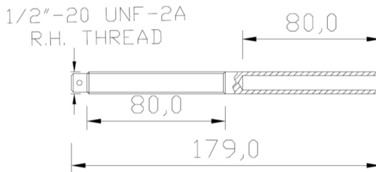
85160-00 Gewindeterminale zum Verpressen (Rechtsgewinde)
