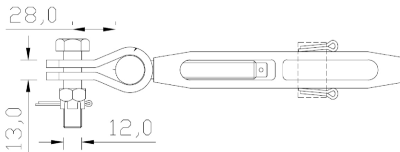
85052-00 Spannhülse mit beweglichem Gabelterminal (Linksgewinde), schmal
