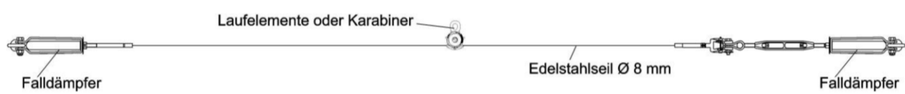
gerades Seilsystem mit zwei Falldämpfern
