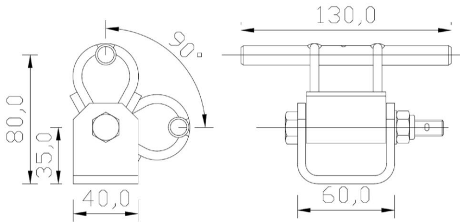
85420-00 schwenkbare Halterung 180°
