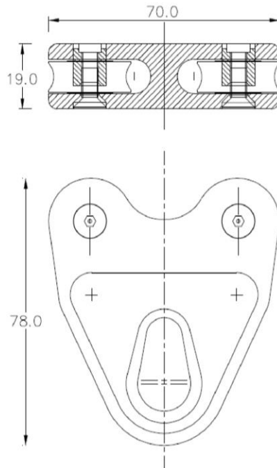
20505-00 beweglicher Anschlagpunkt Single Span
