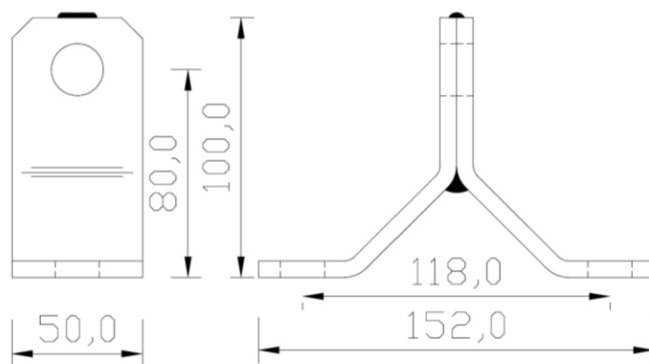
85122-00 Y-Befestigung für Rohrdurchmesser 60 bis 80 mm für 2 x M16
