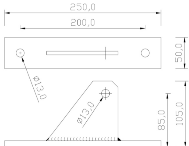
85013-00 Endbefestigung Schwert für 2 x M12, verstärkt
