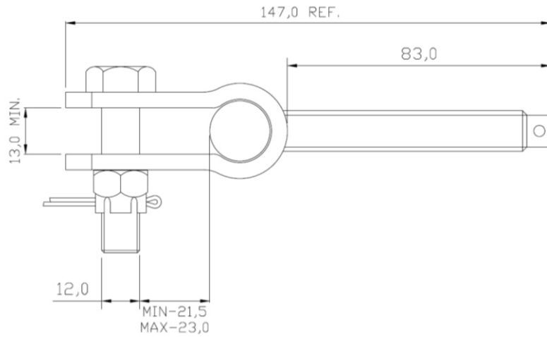
85053-00 bewegliches Gabelterminal für Spannhülse (Rechtsgewinde), breit
