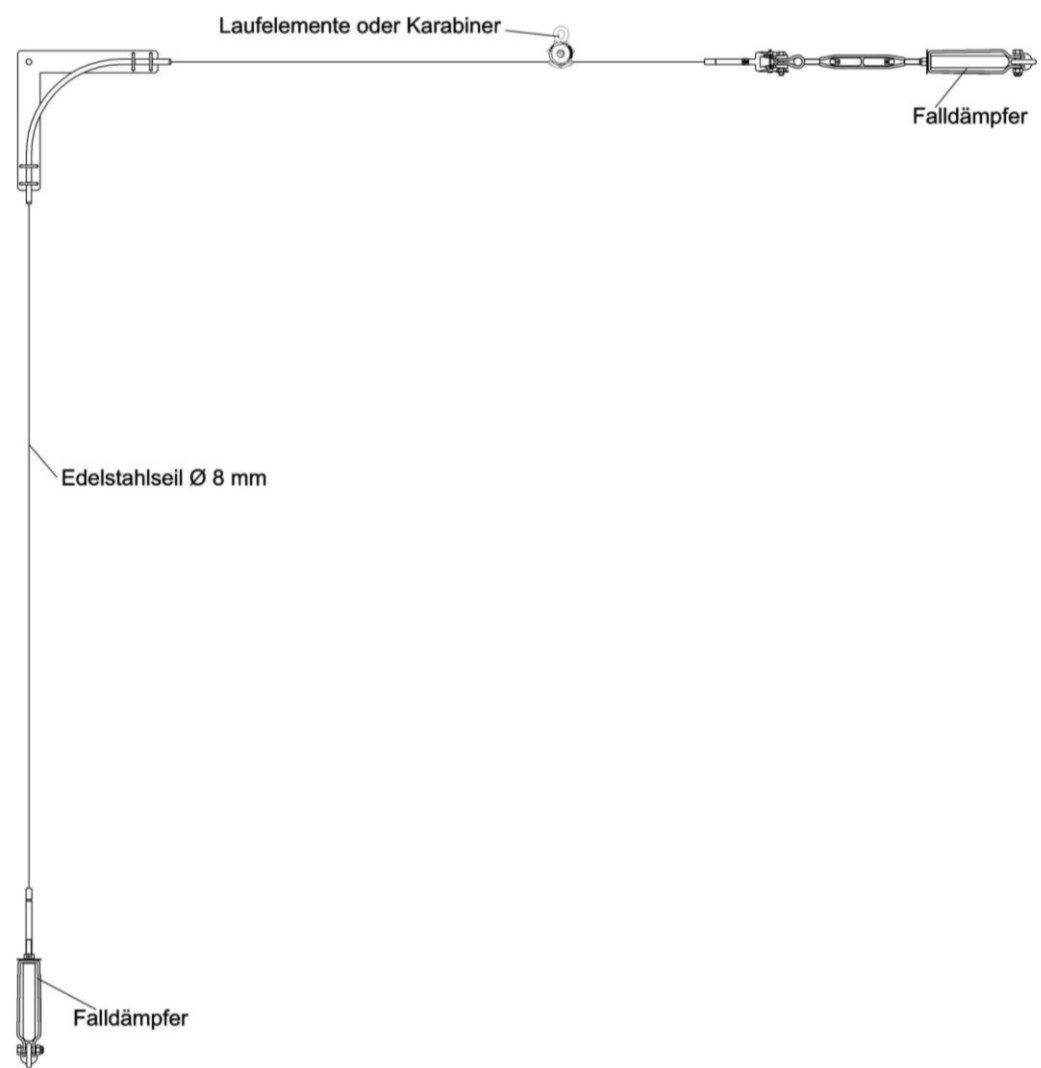
abgewinkeltes Seilsystem mit zwei Falldämpfern
