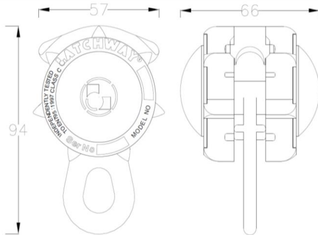
85080-00 beweglicher Anschlagpunkt Standard (Transfastener)
