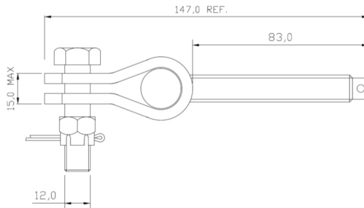
85054-00 bewegliches Gabelterminal für Spannhülse (Rechtsgewinde), schmal
