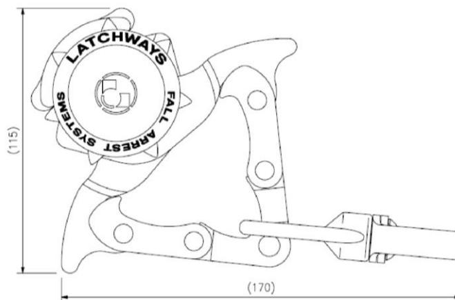
87030-00 mitlaufendes Auffanggerät BridgeLatch bis 70 Grad
