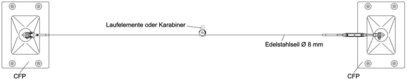
gerades Seilsystem mit Constant Force Posts CFP1 oder CFP2 als Falldämpfer
