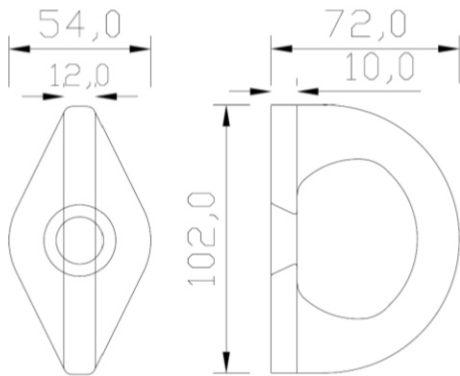
85016-00 Endanker, schwere Ausführung
