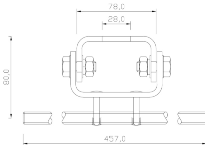
85130-00 variable Halterung (max. 45° pro Seite)
