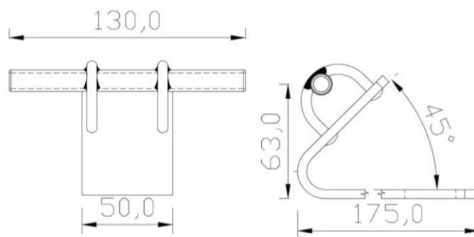
85271-00 45° - Seilhalterung, verlängerte Anschlussplatte
