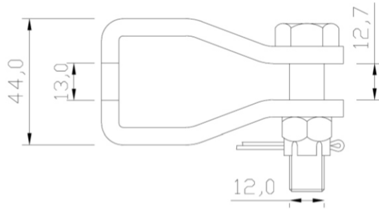
85072-00 Adapter (Gabel)
