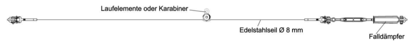
gerades Seilsystem mit einem Falldämpfer
