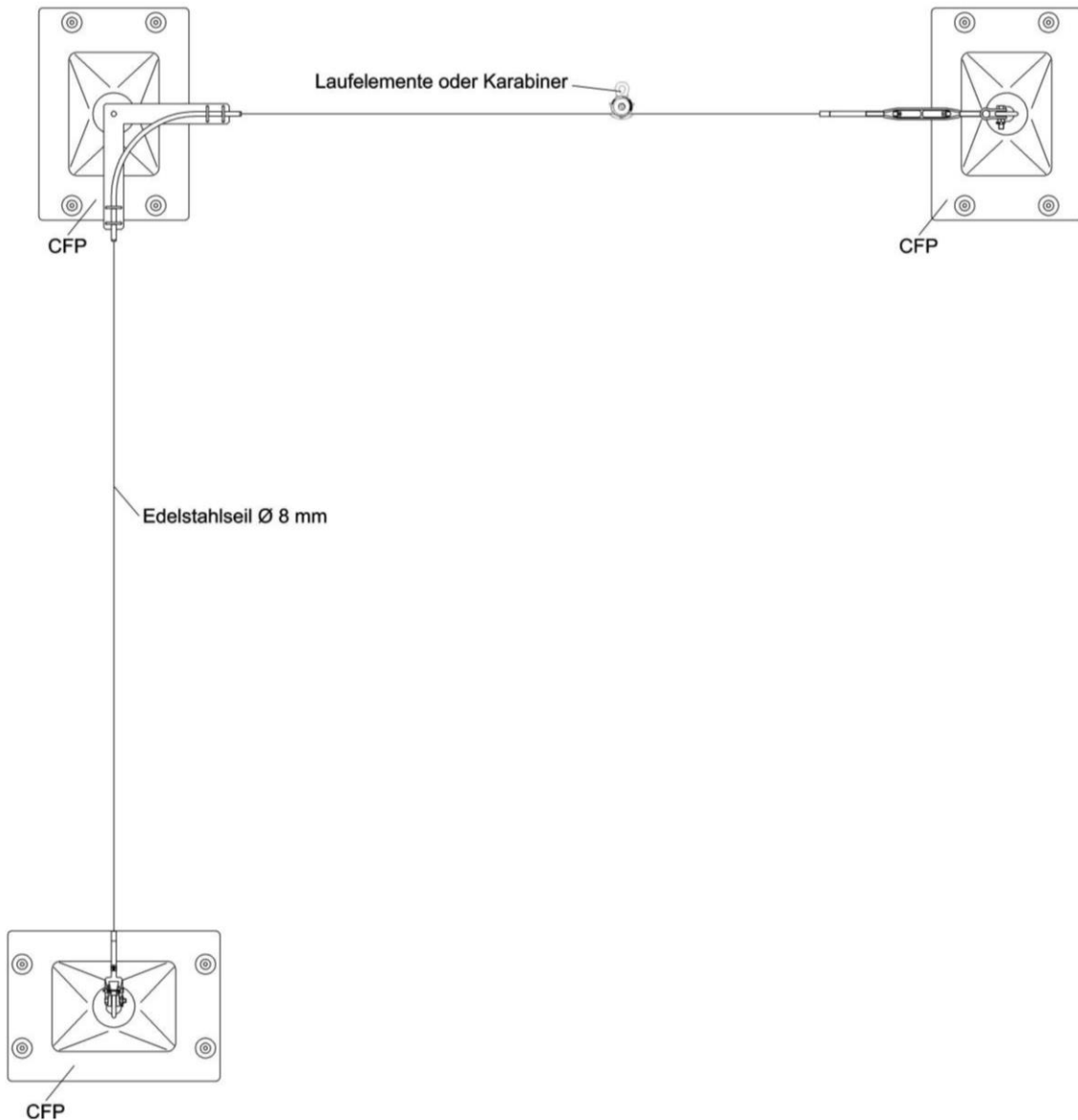
abgewinkeltes Seilsystem mit Constant Force Posts CFP1 oder CFP2 als Falldämpfer Als Zwischenanker können auch Constant Force Posts CFP Int. verwendet werden
