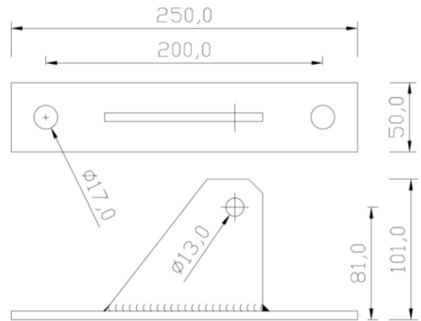
85011-00 Endbefestigung Schwert für 2 x M16
