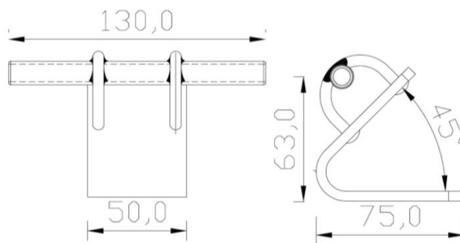
85270-00 45° Seilhalterung
