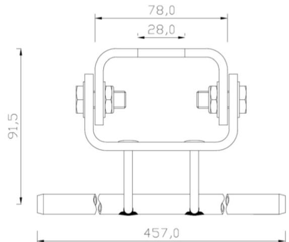
85060-00 Seilhalter für Eckumfahrungen (M12 Verschraubung) mit Spezialgrundplatte
