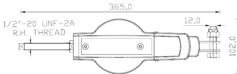
35417-00 6 kN Falldämpfer mit Spulenabsorber mit Gewinde
