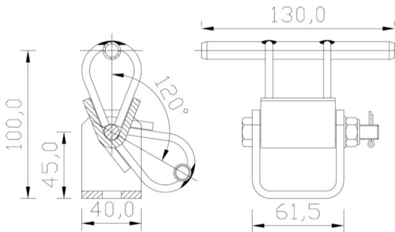
85421-00 schwenkbare Halterung 240°
