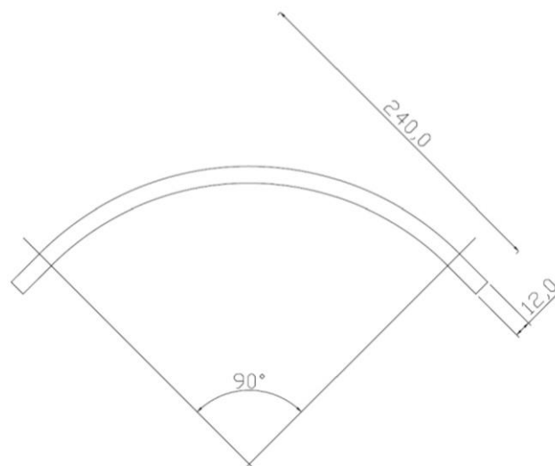
85061-00 Kurvenrohr für 90° - Kurve
