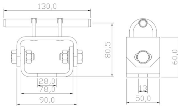
85066-00 Seilhalterung für Eckumfahrung (M12 Verschraubung)
