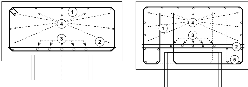
Bild 4: Prinzipielle Bewehrungsführung für die Ausführungsvarianten "mit und ohne Konsoleinspannung"
