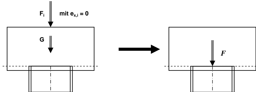
Bild 2: Prinzipielle Darstellung des Lastabtrags "ohne Konsoleinspannung"
