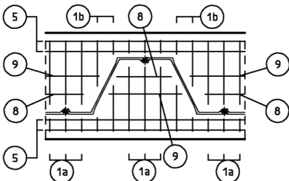
Horizontalschnitt D-D, Untersicht
