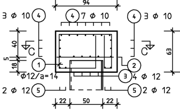
Bügelbewehrung
