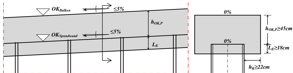
Bild 1b: Schematische Darstellung des Stahlbetonholms mit geneigter Spundwandbohlen-Oberkante, nur in der Ausführungsvariante "mit Konsoleinspannung" möglich
