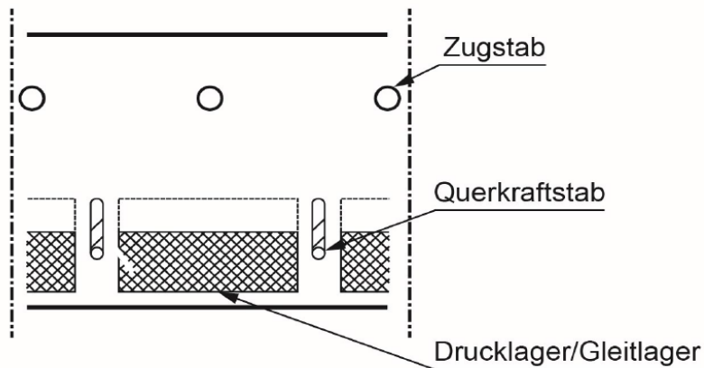
Ansicht Balkenseite
