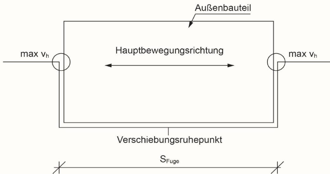
Einbausituation mit Lagerung an gegenüberliegenden Rändern
