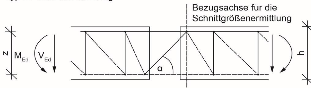
Typ UP indirekte Stützung
