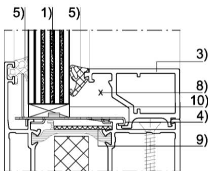
Einbausituation Mono-Verglasung
