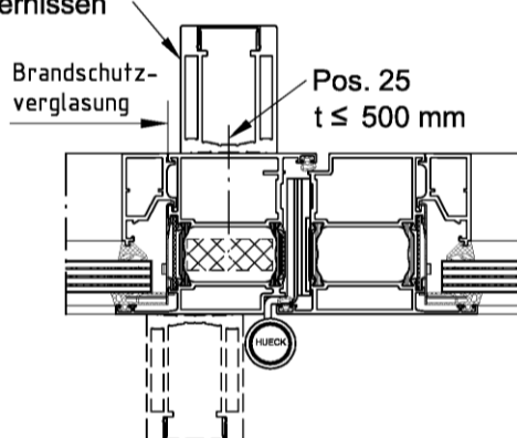
Schnitt D 1
