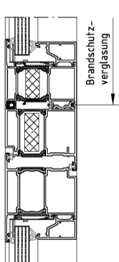
Schnitt E 1
