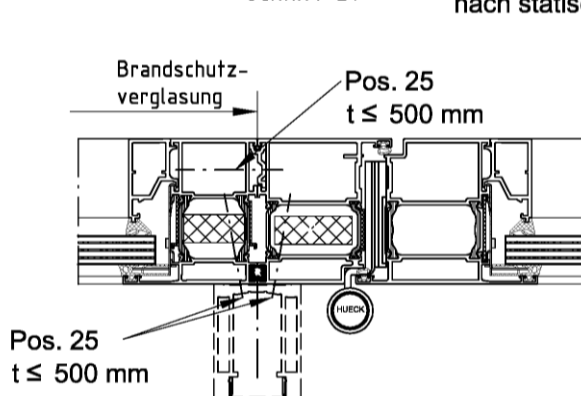
Schnitt D 1
