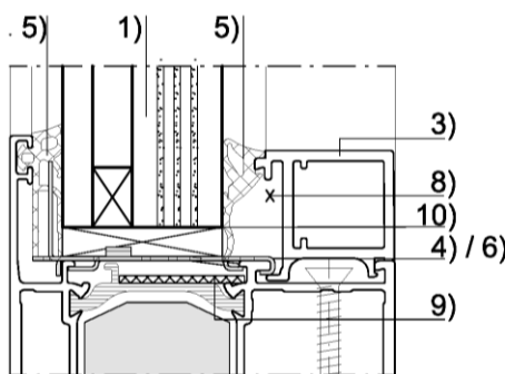
Einbausituation Isolierverglasung
