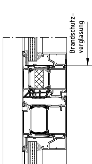
Schnitt E
