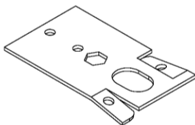
Z 917384 Montagehalter, Edelstahl in Profilmutter eindrehen und mit Senkbohrschraube Z 911050 sichern
