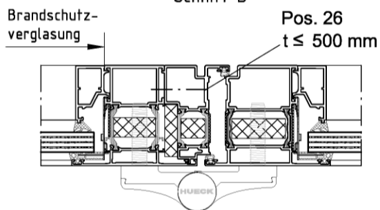
Schnitt D
