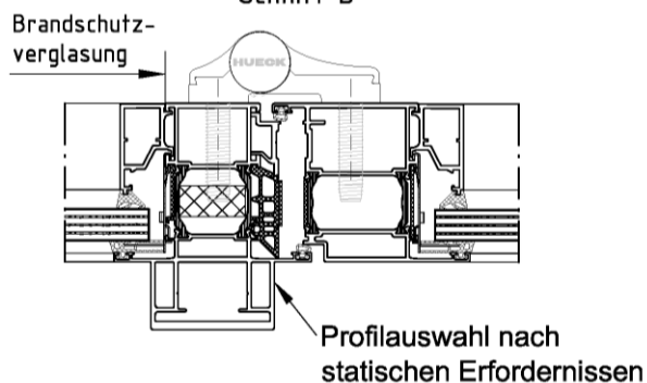
Schnitt D
