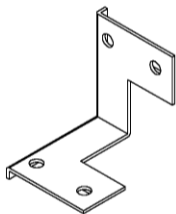
Z 996412 Eckwinkel, Edelstahl für Füllungsgewichte \geq 180 kg
