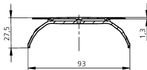
SCHNITT B-B MAßSTAB 1 : 2
