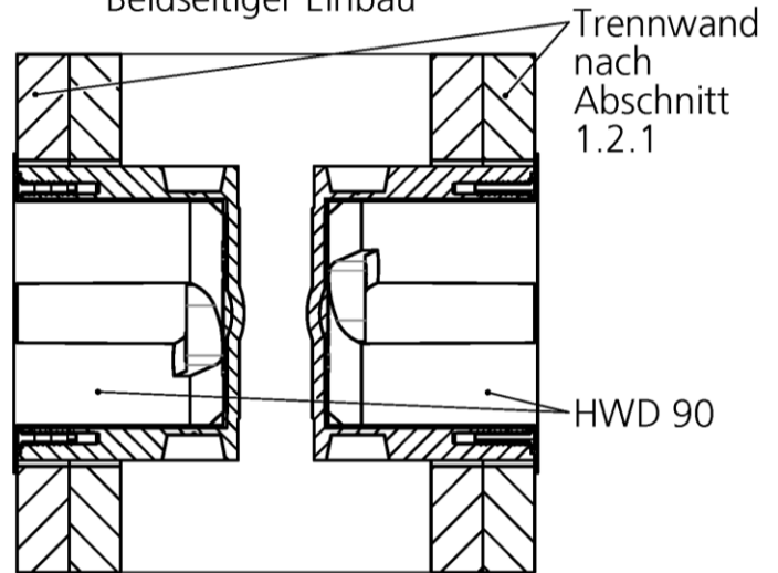
Beidseitiger Einbau Mehrfachanordnung
