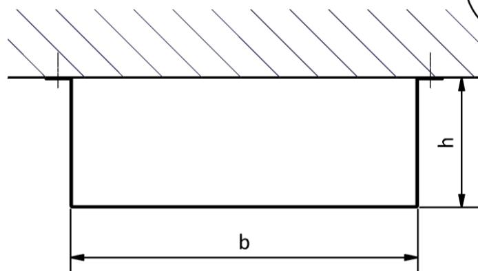
3-seitiger Installationskanal
