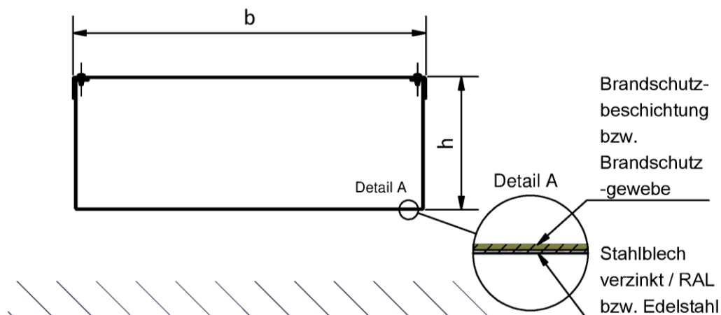
4-seitiger Installationskanal
