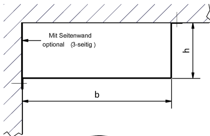
2-seitiger- Installationskanal
