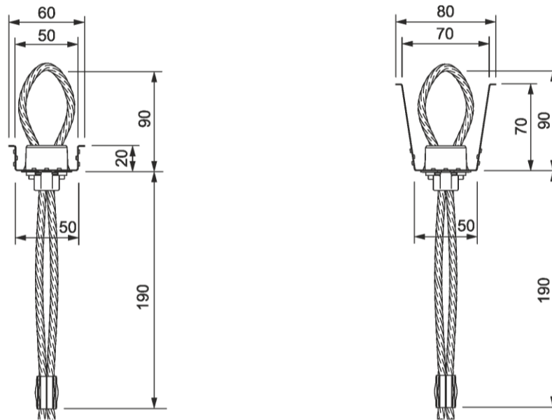
Bild 4: Verwahrkasten mit Seilschleufe – Querschnitt
