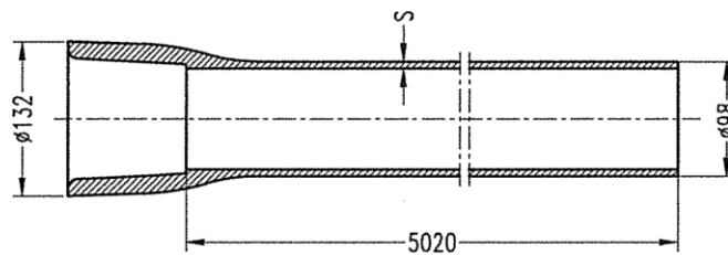
Pfahlrohr \varnothing 98/5000
