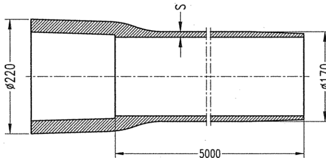
Pfahlrohr \varnothing 170/5000
