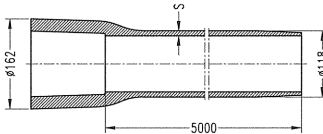
Pfahlrohr \varnothing 118/5000
