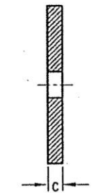
Pfahlkopfplatten Typ B, S 355
