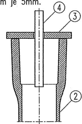
Pfahlkopfplatten Typ B, S 355
