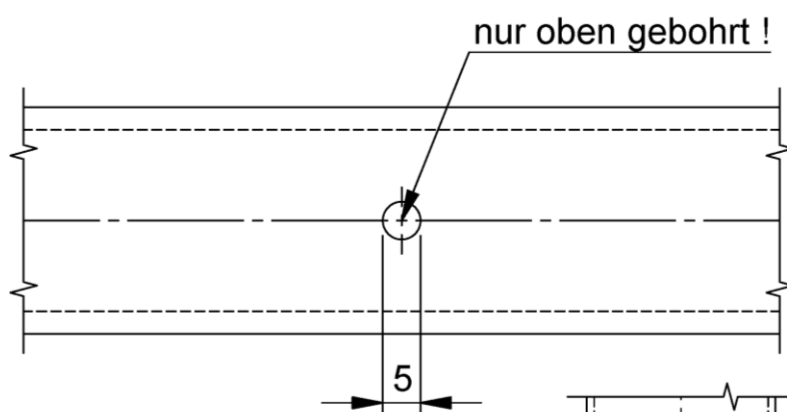
Ansicht X
