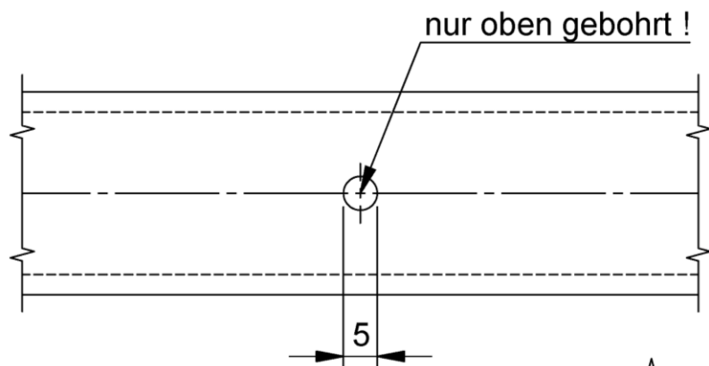
Ansicht X
