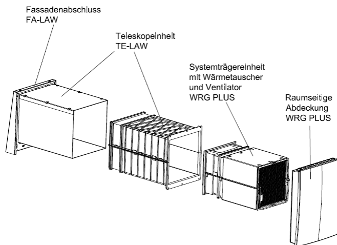
Lüftungsgerät vom Typ "WRG Plus Montagetype LAW"
