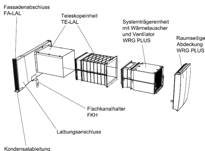
Lüftungsgerät vom Typ "WRG Plus Montagetype LAL"
