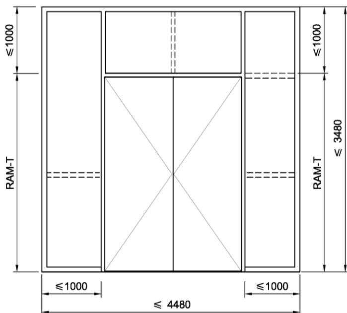
Tür mit Seitenteil(en) / Oberteil
