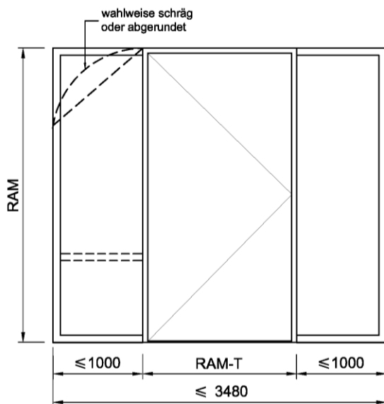
Tür mit Seitenteilen
