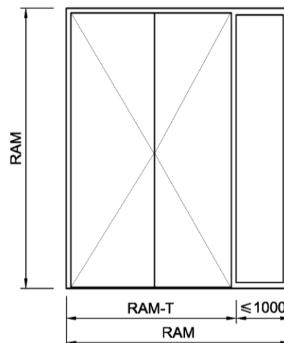
Tür mit Seitenteil
