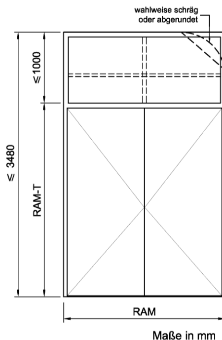
Tür mit Oberteil
