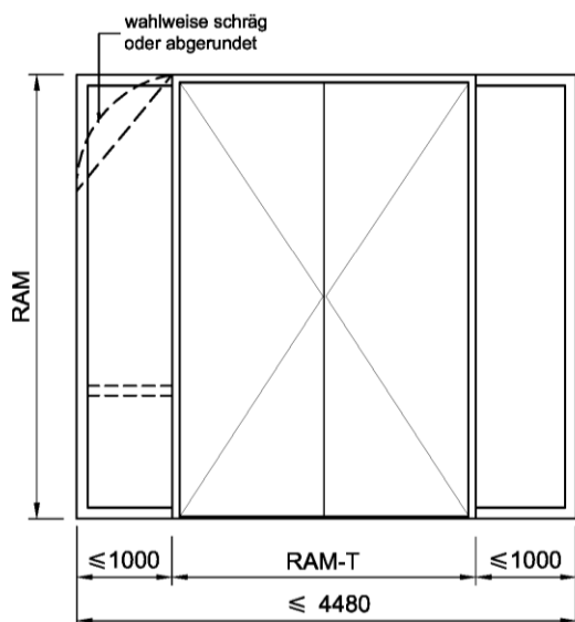
Tür mit Seitenteilen
