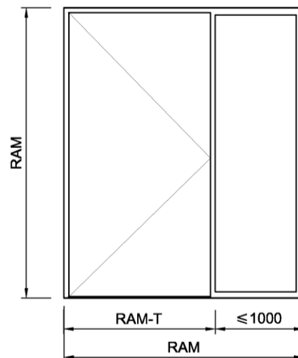
Tür mit Seitenteil
