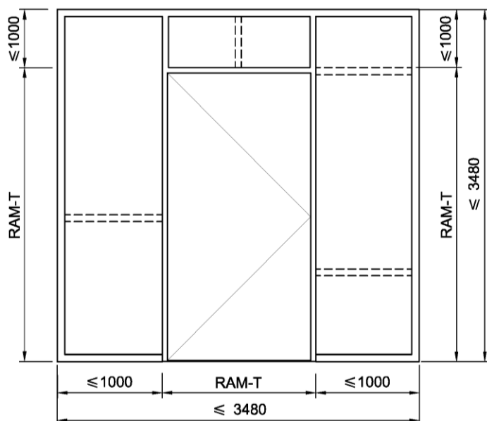
Tür mit Seitenteil(en) / Oberteil
