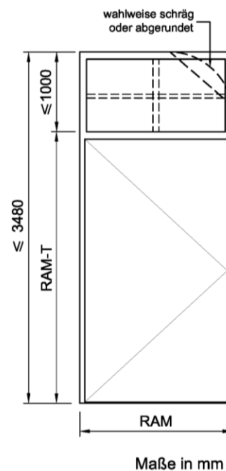
Tür mit Oberteil
