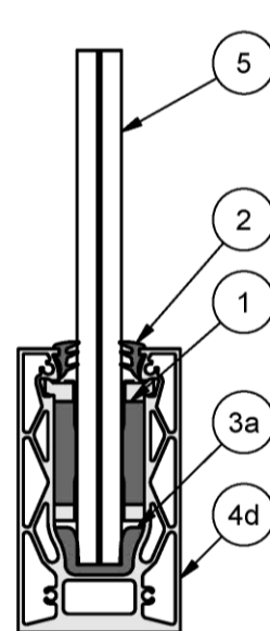
Systemprofil cp1404
