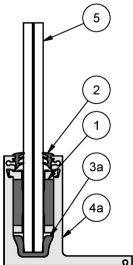
Systemprofil cp1400
