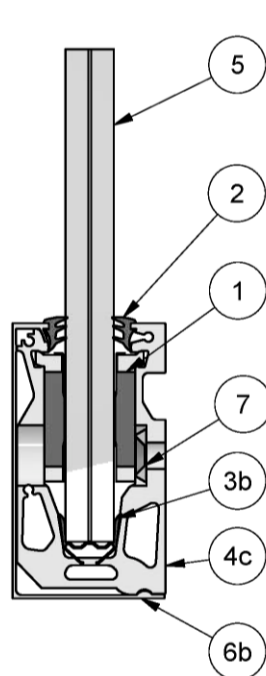
Systemprofil cp1403
