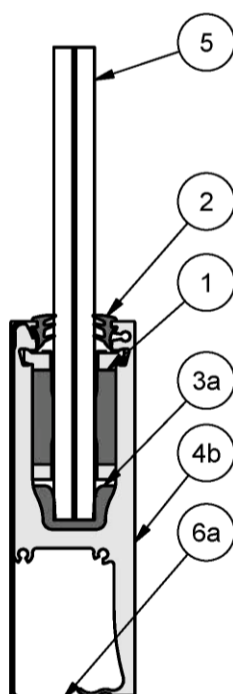
Systemprofil cp1402
