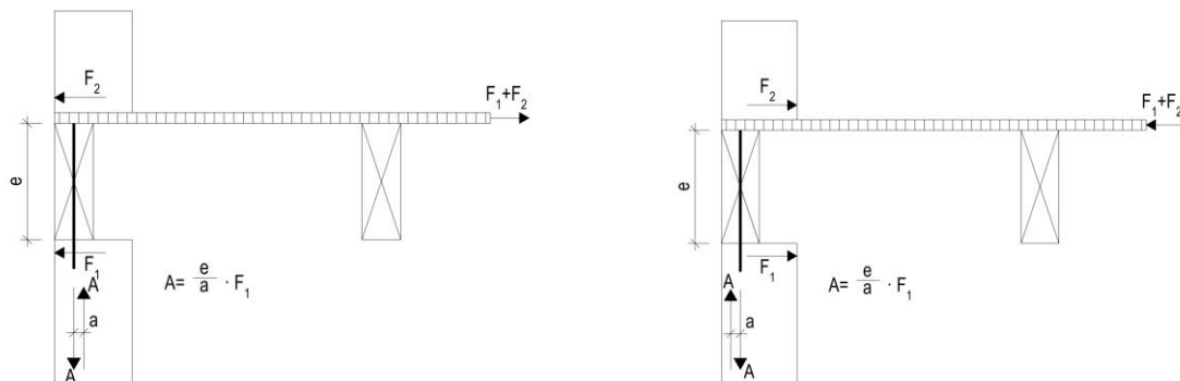
Bild 2 Aufnahme des Versatzmoments infolge Wind durch biegesteifen Anschluss des Randbalkens an die untere Wand
