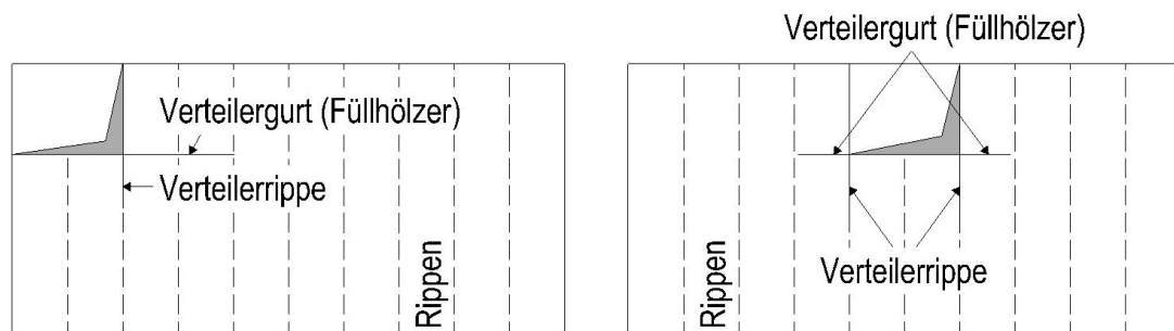
Bild 6 Anordnung von Verteilergurten und -rippen in Verlängerung der Öffnungsränder
