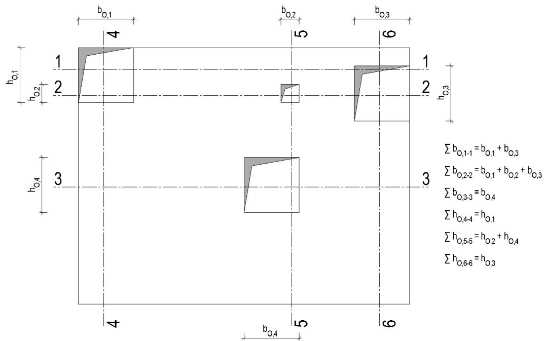
Bild 4 Gleichzeitig zu berücksichtigende Öffnungen in einem Schnitt
