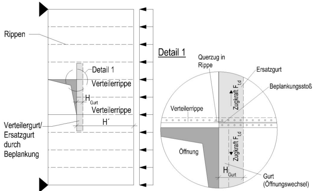
Bild 5 Beplankung als Ersatzgurt/-verteiler für Beanspruchung parallel zu den Rippen
