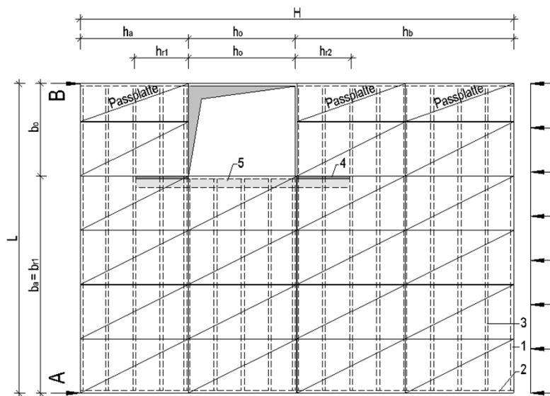
Beanspruchung rechtwinklig zu den Rippen (Anlage 1.2)
