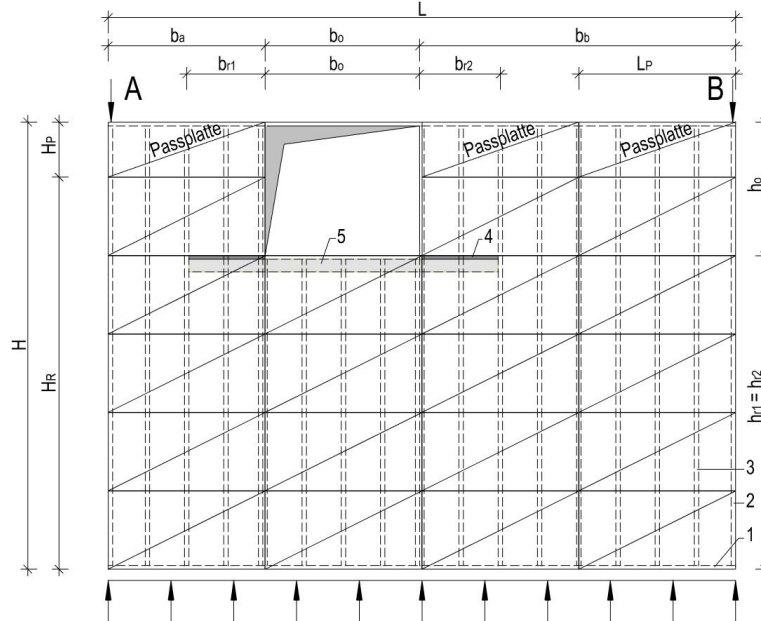
Beanspruchung parallel zu den Rippen (Anlage 1.1)
