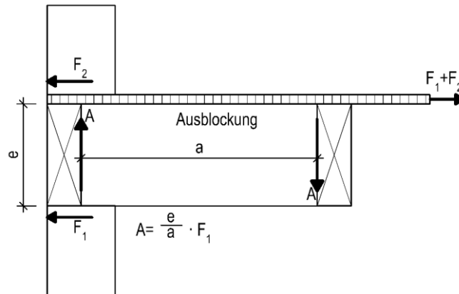
Bild 3 Aufnahme des Versatzmoments durch Ausblockung und Deckenbalken
