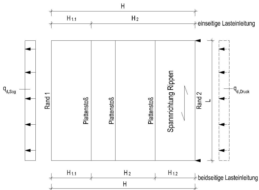
Bild 1 Definition der Scheibenhöhen bei Beanspruchung rechtwinklig zu den Rippen; Bild beispielhaft für Sog an Rand 1 und Druck an Rand 2
