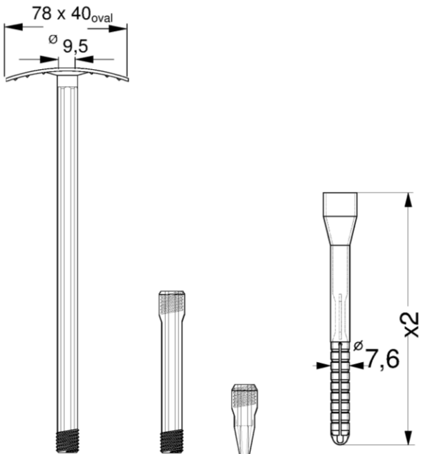
Zahn ZKSH oval Modul 4,8 mit Dübelverlängerung
