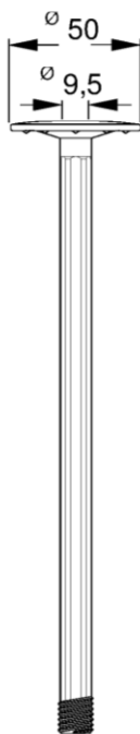
Zahn ZKSH rund Modul 4,8
