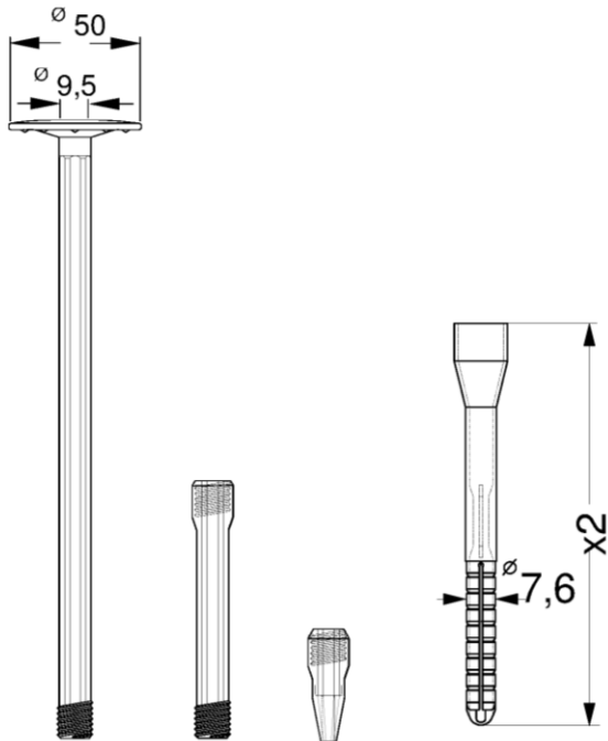
Zahn ZKSH rund Modul 4,8 mit Dübelverlängerung
