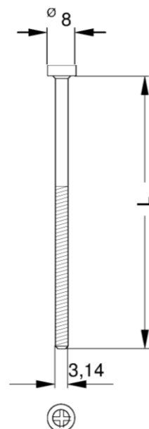
Zahn Metrische Schraube - E 3,14 x L
