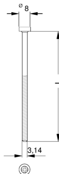
Zahn Metrische Schraube E 3,14 x L
