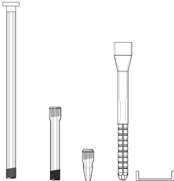
Zahn ZSSB-Modul-Tülle 4,8 mit Modul, Vorsatzdübel und Schiene
