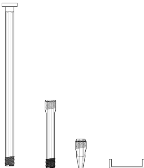
Zahn ZSSB-Modul-Tülle 4,8 mit Modul und Schiene
