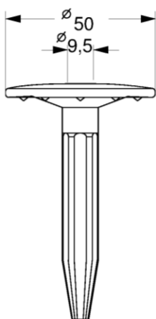
Zahn ZKSH rund
