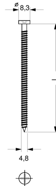
Zahn ZDBK Dübel 4,8 x L
