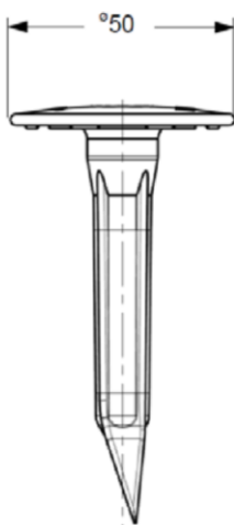
Zahn ZKSH-Rplus Pfahlspitze
