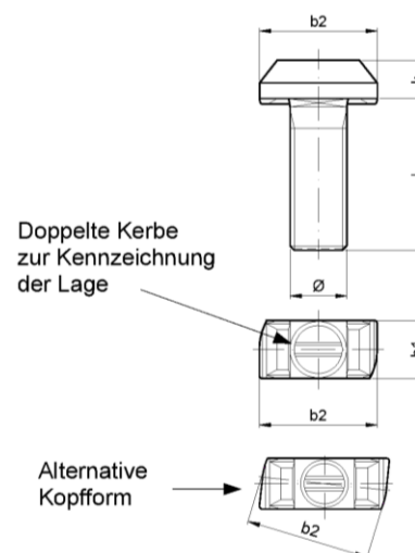
Bild 3 - Doppelkerbzahnschraube
