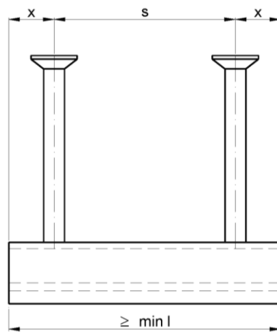
Bild 3 Anschweißanker rund
