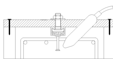
c) an der Bauteiloberseite
