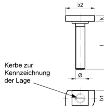
Bild 2 - Hakenkopfschraube
