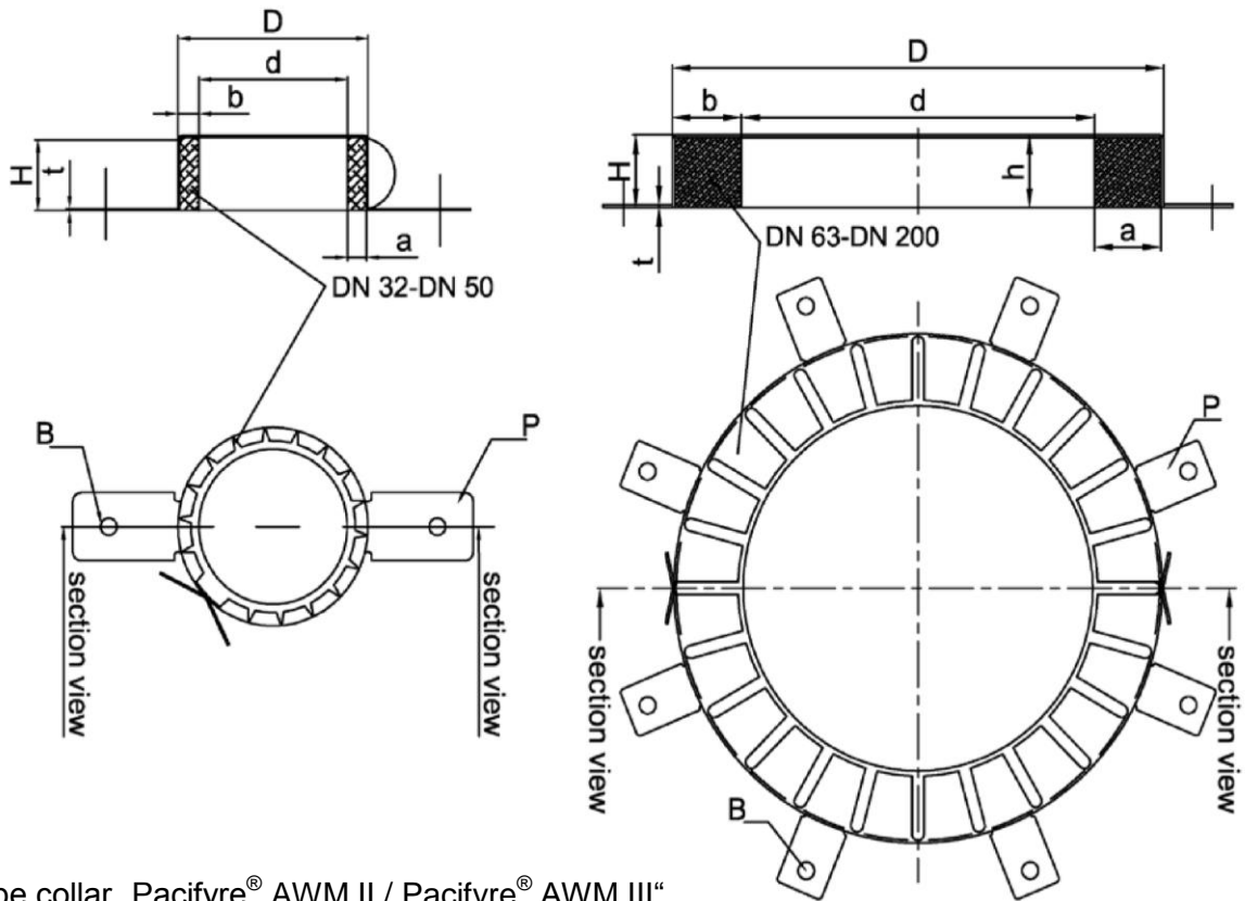
Pipe collar „Pacifyre® AWM II / Pacifyre® AWM III“ in the dimensions AWM II
