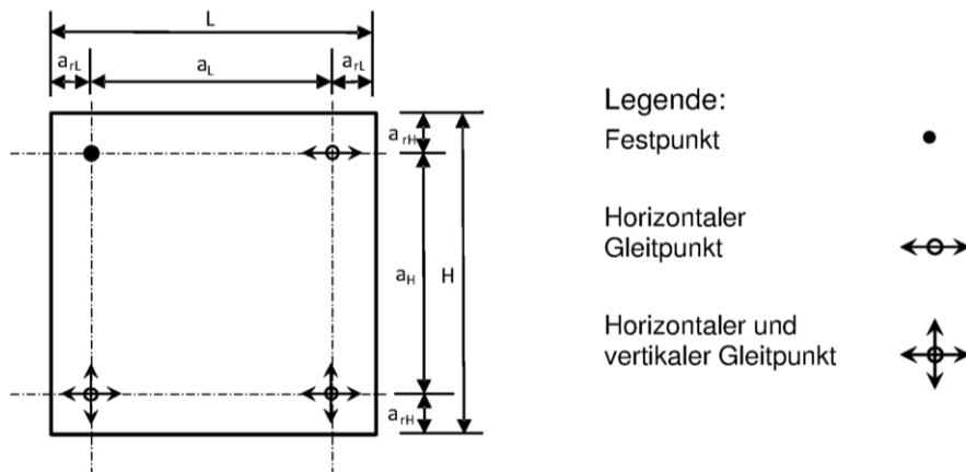
Bild B1: Geometrie der Natursteinplatten
