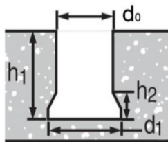
Bild B1: Bohrlochgeometrie
