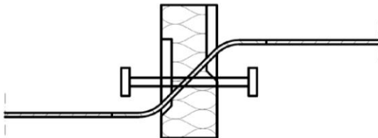
Fig. 3 Schöck Isokorb® type Q
