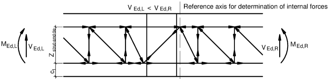
Fig. 29 Schöck Isokorb® type D
