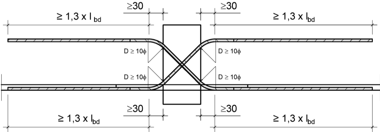
Fig. 31 Schöck Isokorb® type D
