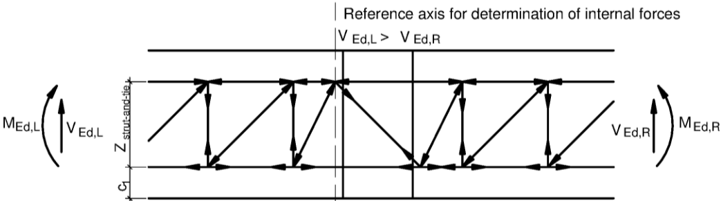
Fig. 28 Schöck Isokorb® type D
