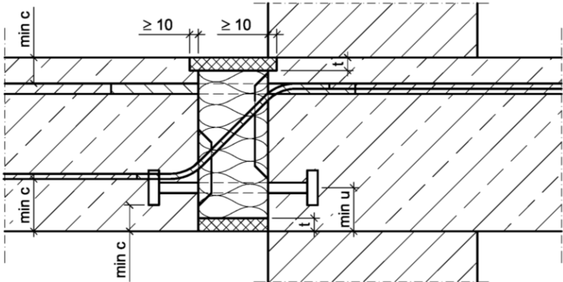
Fig. 21 Schöck Isokorb® type K und type KF with SCE
