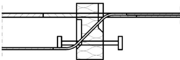
Fig. 1 Schöck Isokorb® type K
