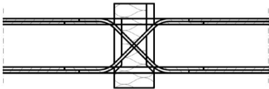
Fig. 5 Schöck Isokorb® type D
