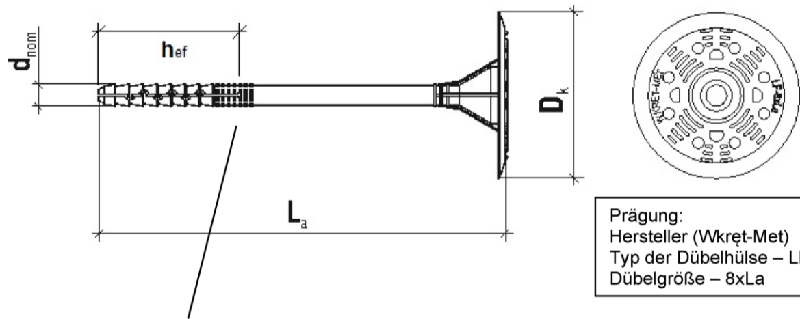
Markierung der Verankerungstiefe
