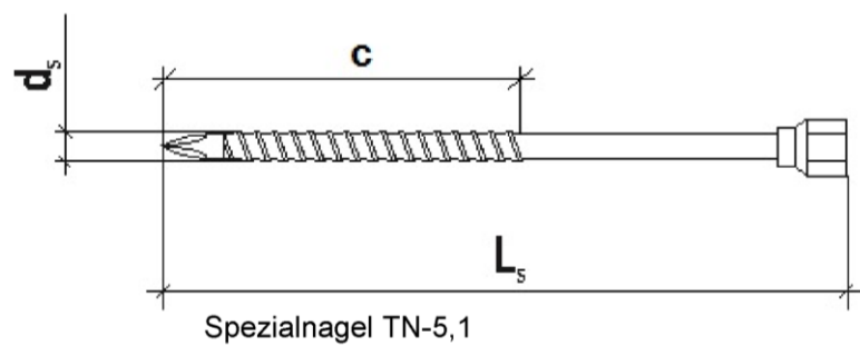
Markierung der Verankerungstiefe
