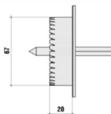
Spezialwerkzeug WK-FT für die tiefergesetzte Montage
