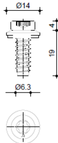
Gewindefurchende Schraube JZ3-6.3x19-E14
