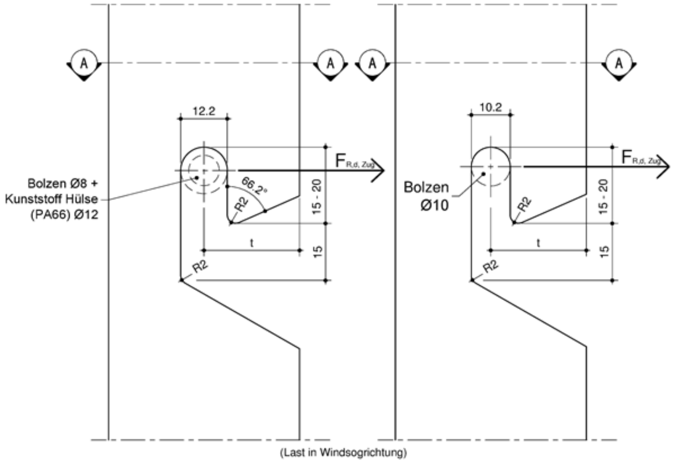
Variante A - Ø8mm Bolzen und Kunststoffhülse Ø12mm
