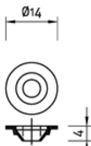
Material: TPE, Härte ShoreD: 35 nach DIN ISO 7619
