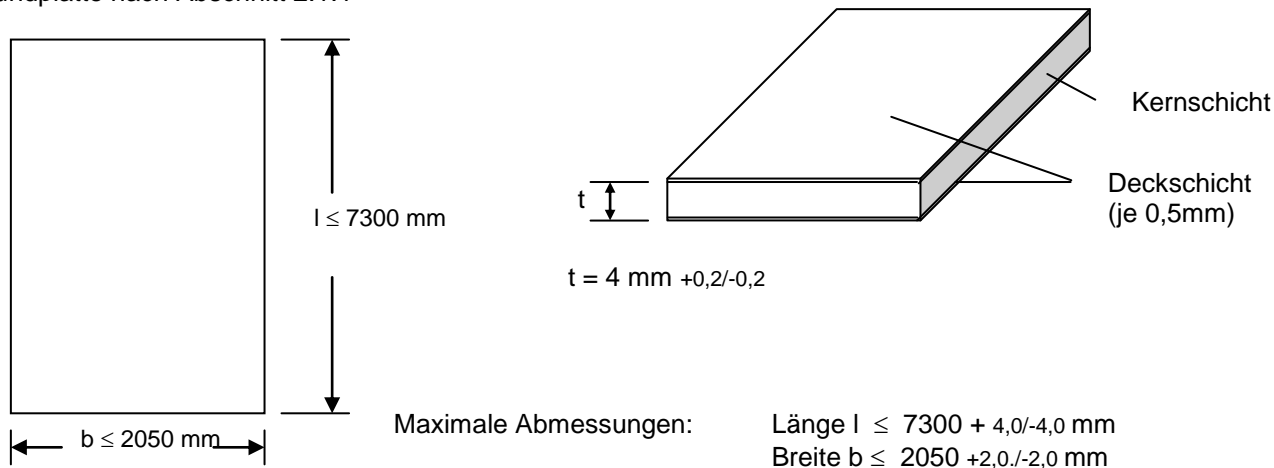
Verbundplatte nach Abschnitt 2.1.1
