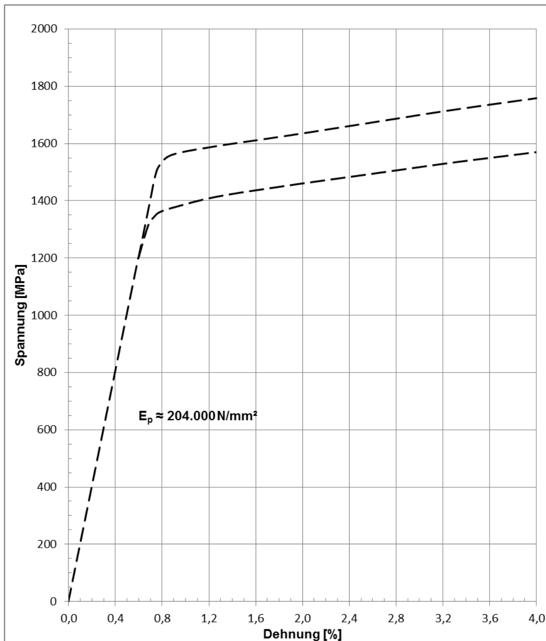
Bild 2: Prinzipieller Spannungs-Dehnungs-Verlauf
