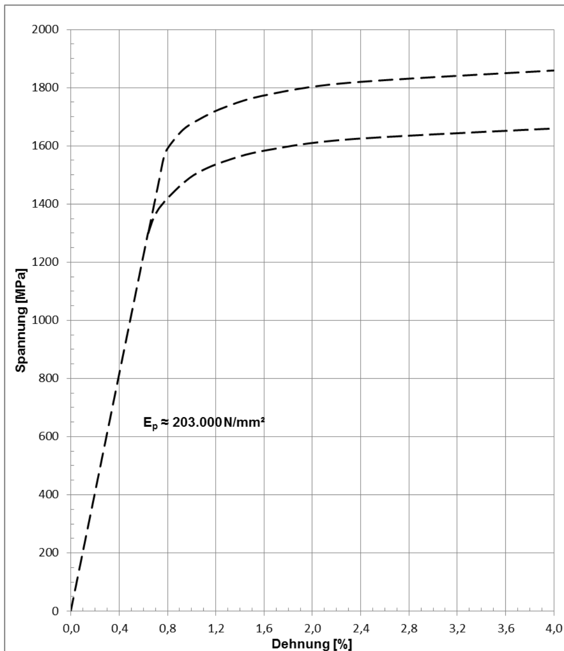
Bild 2: Prinzipieller Spannung-Dehnungs-Verlauf
