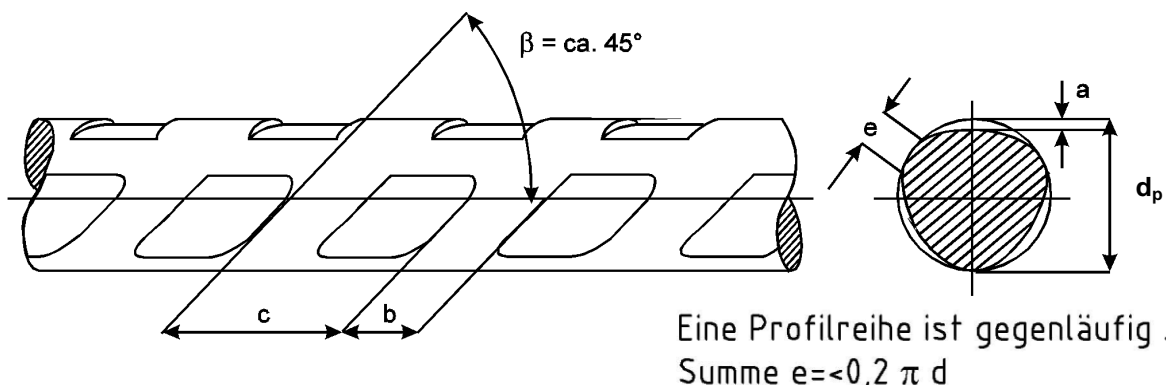
Bild 1: Ansicht des profilierten Spannstahldrahts
