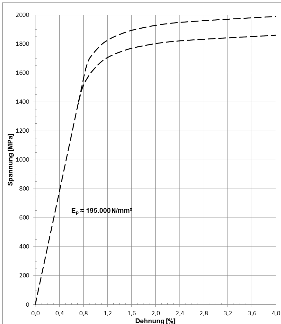
Bild 2: Prinzipieller Spannung-Dehnungs-Verlauf
