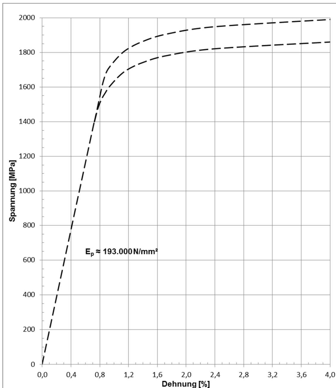
Bild 2: Prinzipieller Spannungs-Dehnungs-Verlauf
