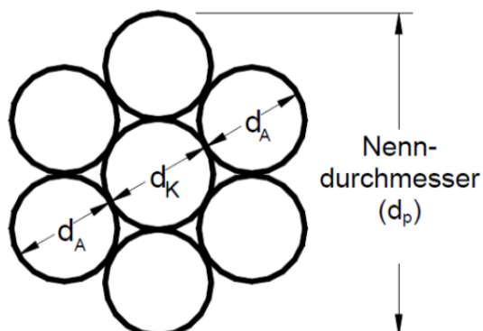
Bild 1: Darstellung des Spannstahlilitzen-Querschnitts
