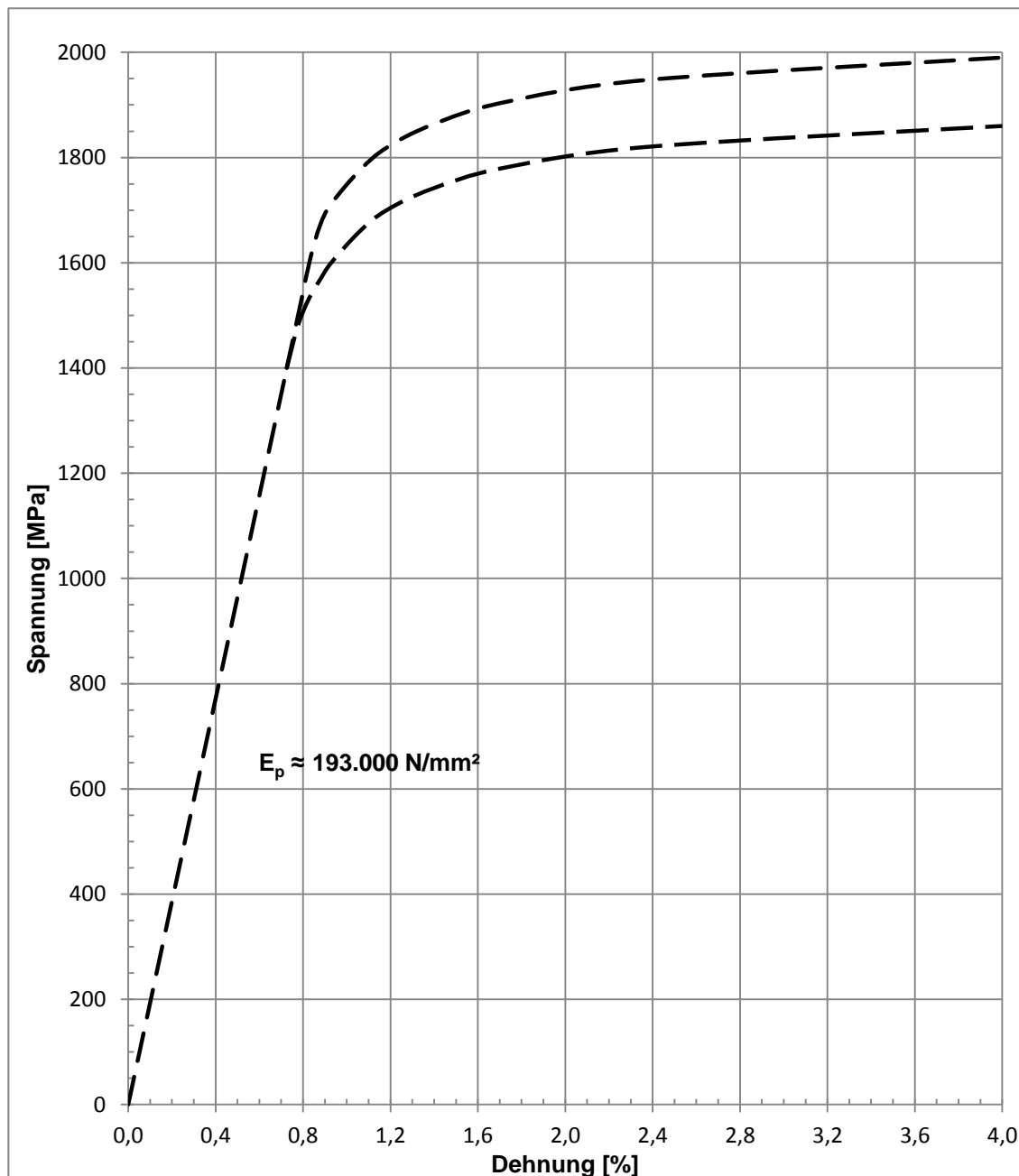
Bild 2: Prinzipieller Spannung-Dehnungs-Verlauf
