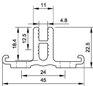
Aufsatzkanal aus Aluminium AK 5010
