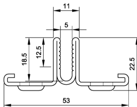
Aufsatzkanal aus Stahl AK 6020
