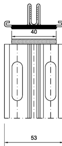
Querschweißung
