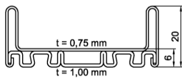
DL 5044, Edelstahl
