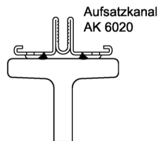
z.B. Stahl-Walzprofil
