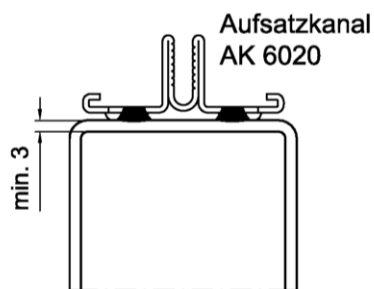
Stahl-Hohlprofile
