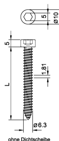
ohne Dichtscheibe
