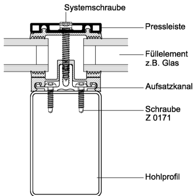
Schichtbare versenkte Verschraubung
