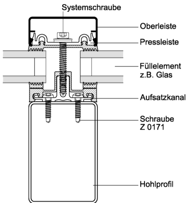
Verdeckte Verschraubung
