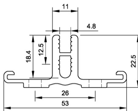
Aufsatzkanal aus Aluminium AK 6010
