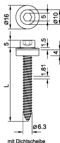
mit Dichtscheibe
