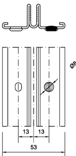
Schweißung im Rund- loch Ø 8 mm
