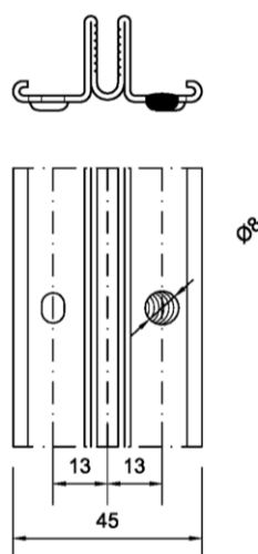
Schweißung im Rund- loch Ø 8 mm
