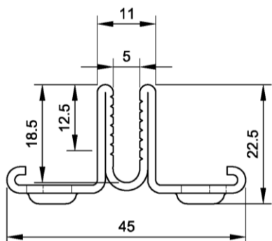
Aufsatzkanal aus Stahl AK 5020
