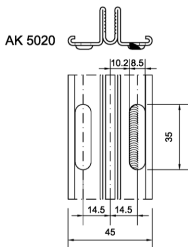
Schweißung im Lang- loch 8,5 x 35 mm
