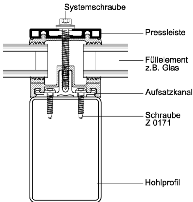
Schichtbare Verschraubung
