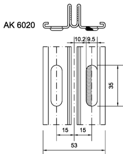
Schweißung im Lang- loch 8,5 x 35 mm
