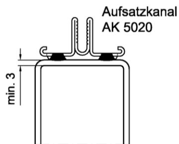
Stahl-Hohlprofile
