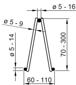
Bild 2: E-Gitterträger
