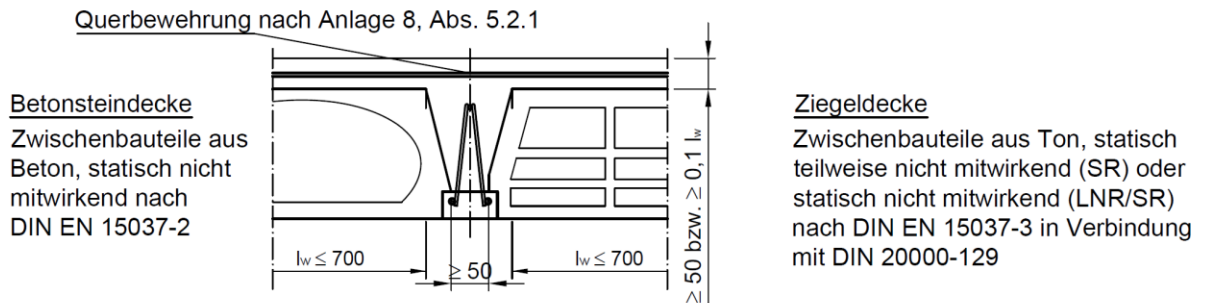
Bild 8: Rippendecke nach Anlage 8, Abschnitt 5
