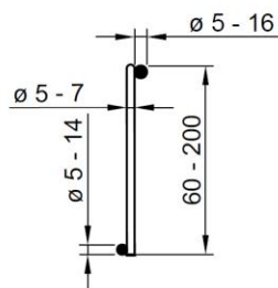
Bild 3: DH-Gitterträger
