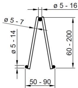
Bild 1: D-Gitterträger
