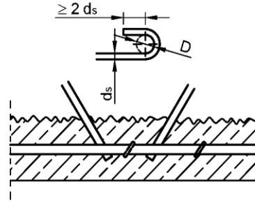
Bild 14: Querbügel
