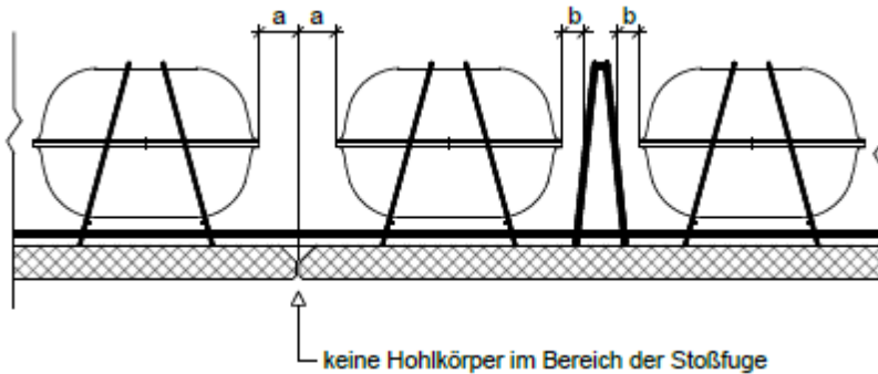
Bild 4: Mindestabstände der Cobiax Slim-Line-Einbauelemente
