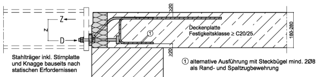
Abb. 26: Schöck Isokorb® Typ QS8, QS10 und QS12
