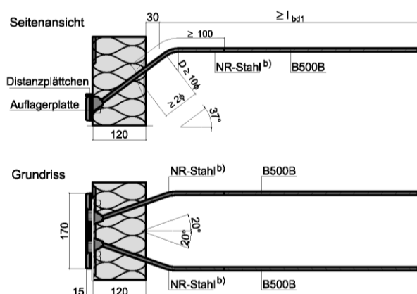
Abb. 35a bis 35d: Querkraftstäbe 2 Ø d inkl. Auflagerplatte
