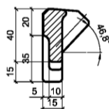
Abb. 52: Auflagerplatte
