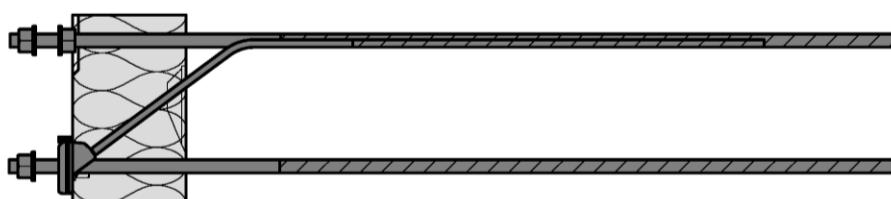
Abb.6 Schöck Isokorb® Typ KSXT14 VV
