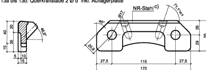
Abb. 14: Auflagerplatte
