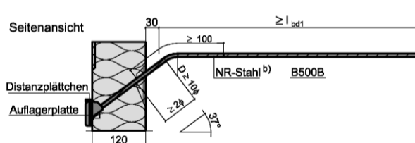
Abb. 50: Drucklager 2 Ø 14
