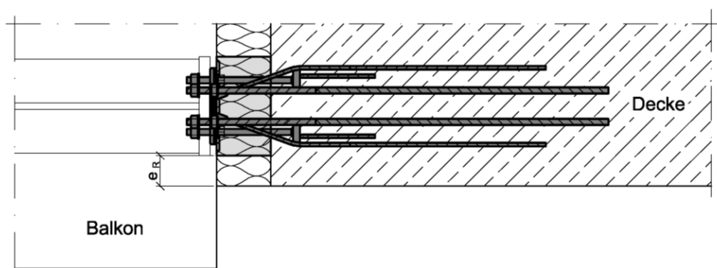
Abb. 77 randnahe Einbau
