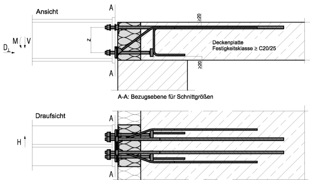
Abb. 65 und 66: Schöck Isokorb® Typ KSXT14 V8, Schnittgrößendefinition
