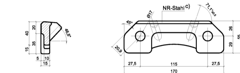
Abb. 36: Auflagerplatte
