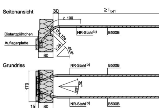
Abb. 24a bis 24d: Querkraftstäbe 2 Ø d inkl. Auflagerplatte
