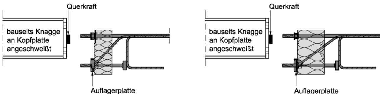
Abb. 79 Querkraftübertragung durch Knappe
