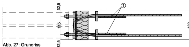
Abb. 27: Grundriss
