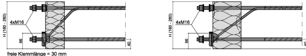
Abb. 81 Seitenansicht: Schöck Isokorb® Typ KS14 VV und Typ KSXT14VV
