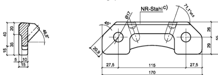
Abb. 19: Auflagerplatte
