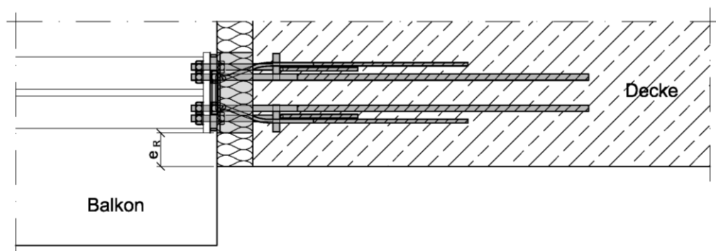
Abb. 63 randnahe Einbau
