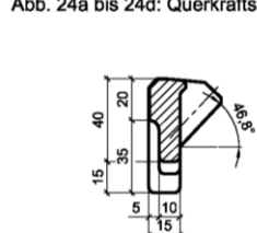
Abb. 25: Auflagerplatte
