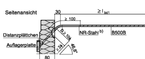
Abb. 11: Zugstäbe 2 \varnothing 14
