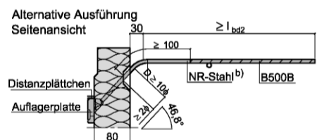
Abb. 12: Drucklager 2 \varnothing 14
