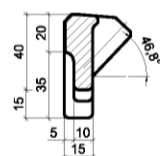
Abb. 41: Auflagerplatte
