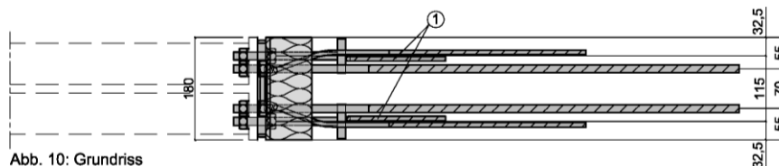
Abb. 10: Grundriss
