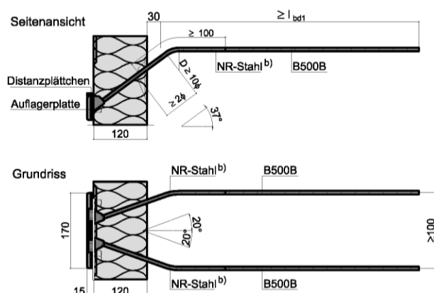
Abb. 40a bis 40d: Querkraftstäbe 2 Ø d inkl. Auflagerplatte
