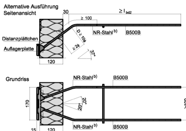
Abb. 34: Drucklager 2 Ø 14
