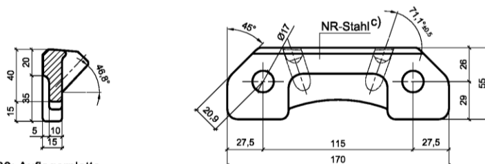
Abb. 30: Auflagerplatte
