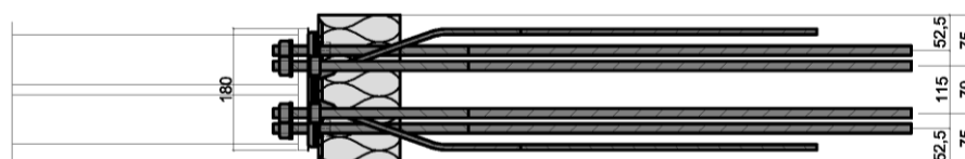
Abb. 38: Grundriss
