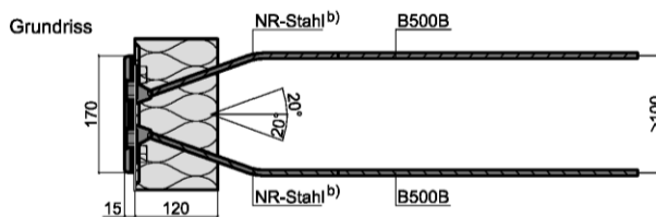
Abb. 51a bis 51d: Querkraftstäbe 2 Ø d inkl. Auflagerplatte
