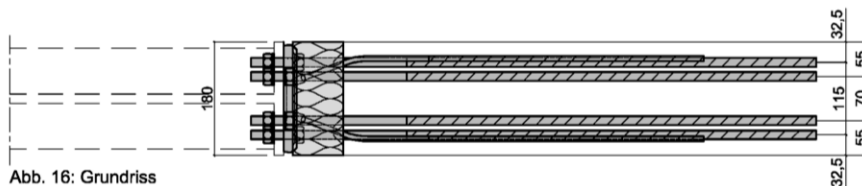
Abb. 16: Grundriss
