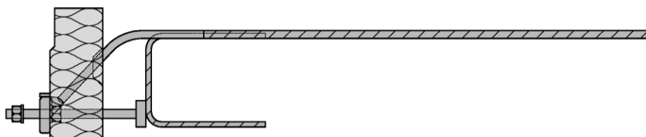
Abb.4 Schöck Isokorb® Typ QS8, QS10 und QS12
