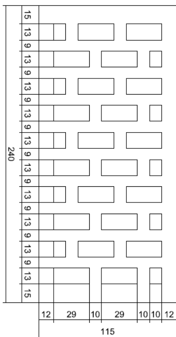
Abbildung 8: Hochlochziegel (Hlz) I
