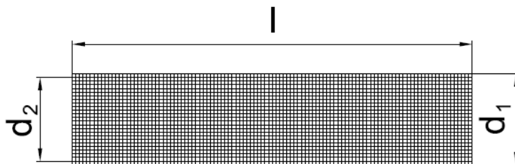
Abbildung 6: Siebhülse SH 25
