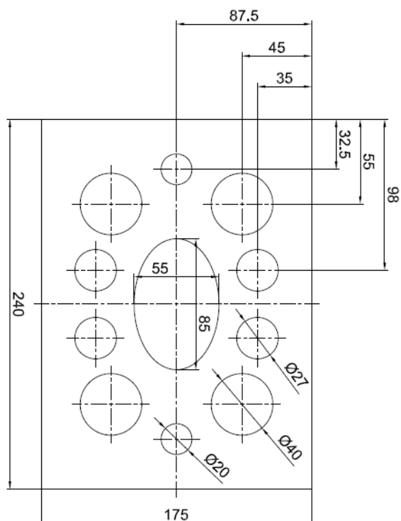
Abbildung 10: Kalksandlochstein (KSL)
