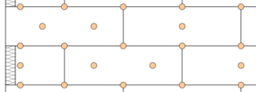
8 Dübel / m 2
