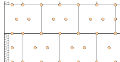
9 Dübel/m 2
