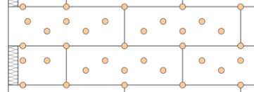
15 Dübel / m 2
