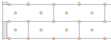
9 Dübel / m 2
