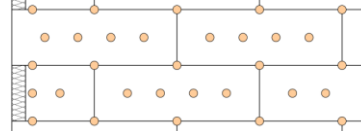
13 Dübel / m 2
