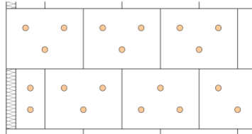
6 Dübel/m 2
