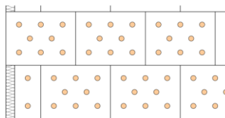
16 Dübel / m 2
