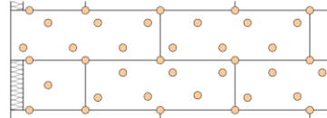
16 Dübel / m 2
