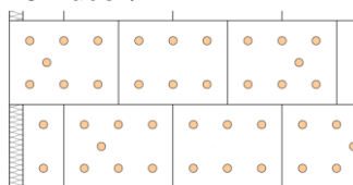
14 Dübel / m 2
