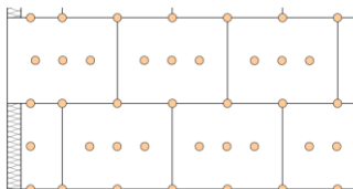
11 Dübel / m 2
