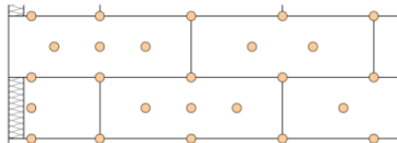
10 Dübel / m 2
