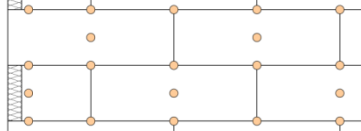
7 Dübel / m 2
