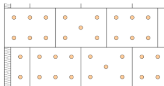
12 Dübel / m 2
