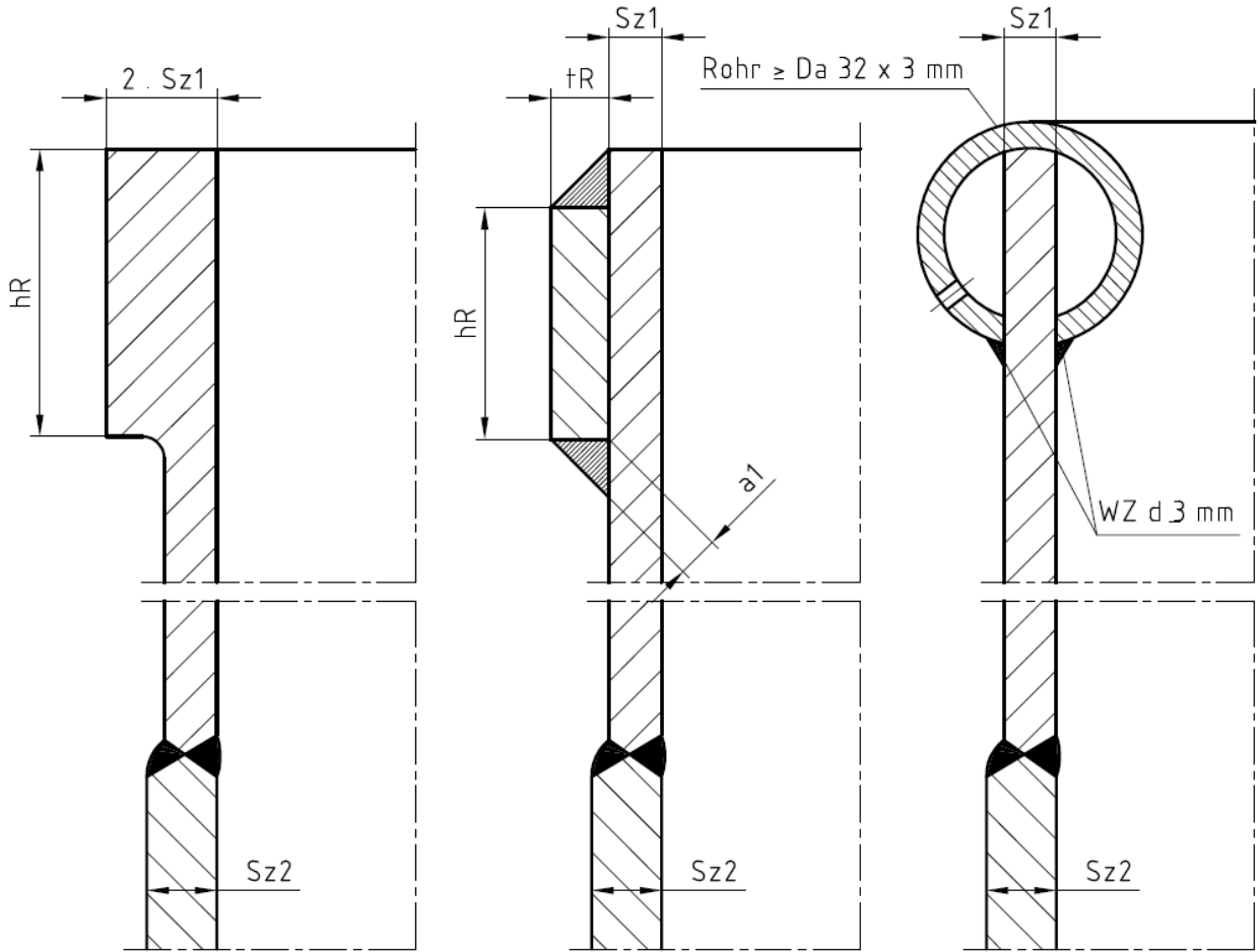
mit Verstärkungs- ring
