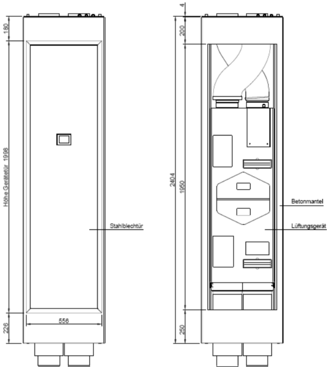
Das Lüftungsgerät "AERA EQONIC Premium" wird im "AERA EQONIC Modulkörper", bestehend aus einem Betonmantel und einer Stahltür, installiert.
