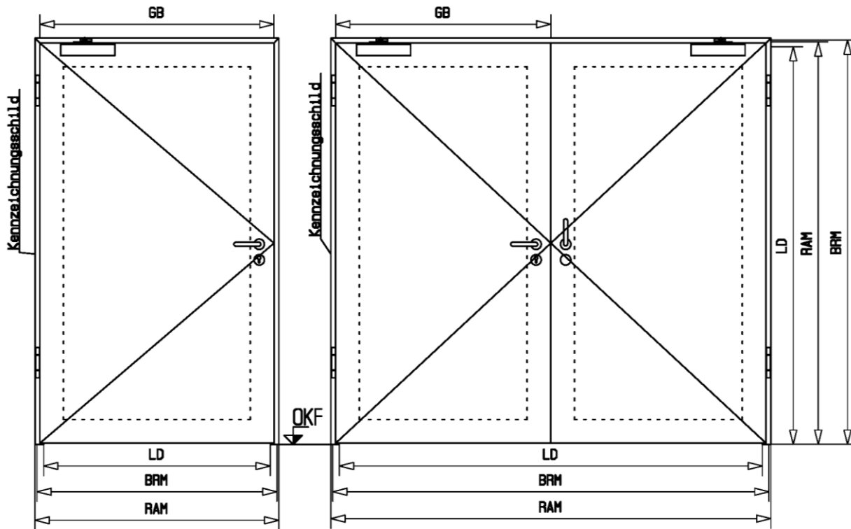
dargestellt: Gangflügel DIN links Gangflügel DIN rechts im Spiegelbild
