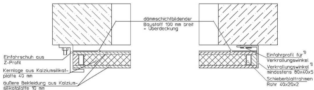
Schnitt B-B aus Anlage 4
