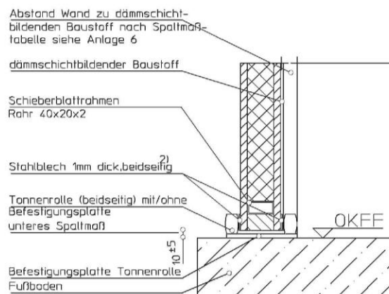
Detail A'' aus Anlage 6
