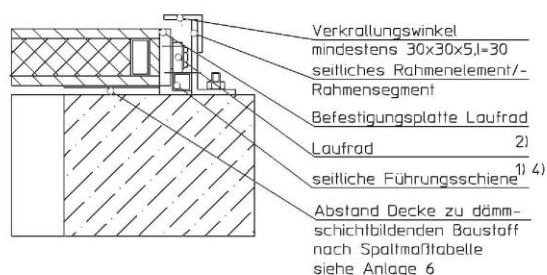
Detail B aus Anlage 5
