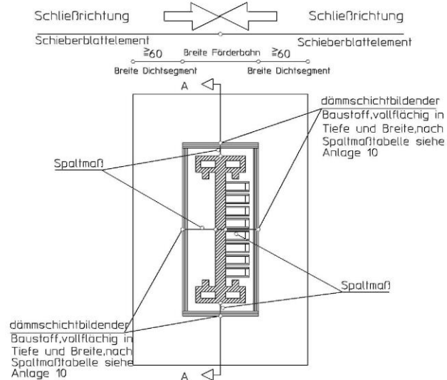
Vorderansicht Elektrohängebahn
