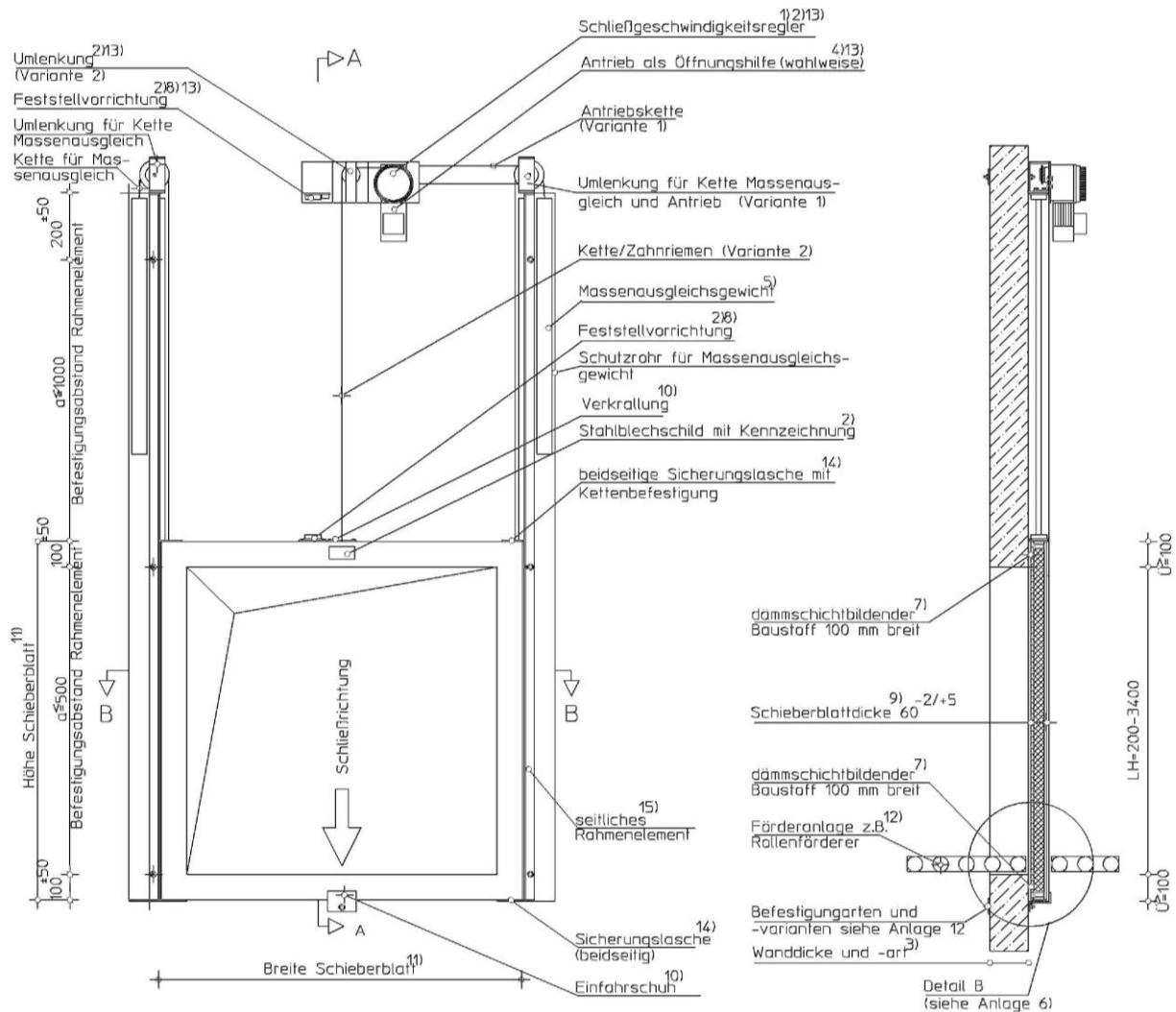
Vorderansicht
