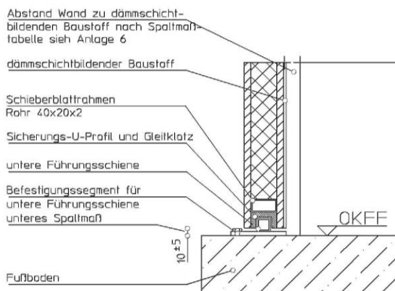
Detail A' aus Anlage 6
