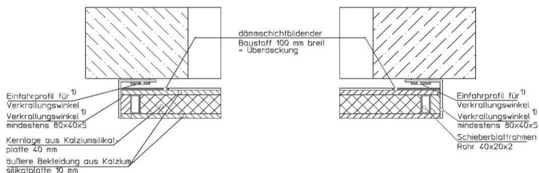
Detail A' aus Anlage 6
