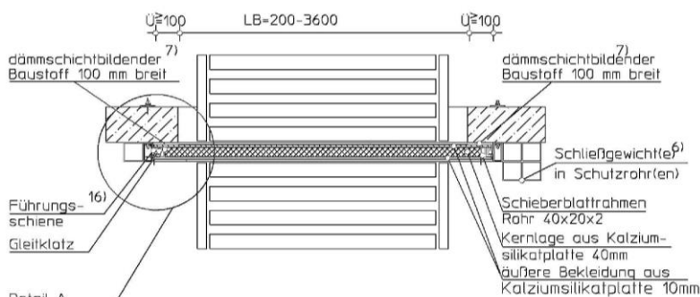
Schnitt B-B
