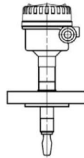
Flanschmontage (Standardlänge)
