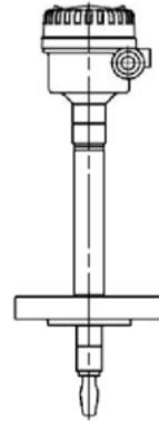
Flanschmontage (Standardlänge)
