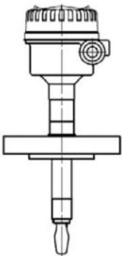
Flanschmontage (mit Verlängerung)
