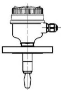
Flanschmontage (Standardlänge)
