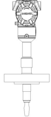
Flaschmontage (mit Standardlänge)
