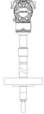
Flaschmontage (mit Standardlänge)
