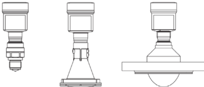
VEGAPULS 64
