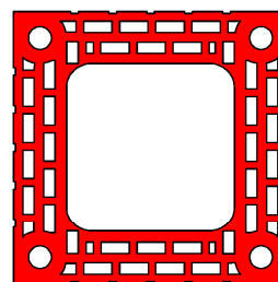
Ziegelaußenschale ungedämmt
