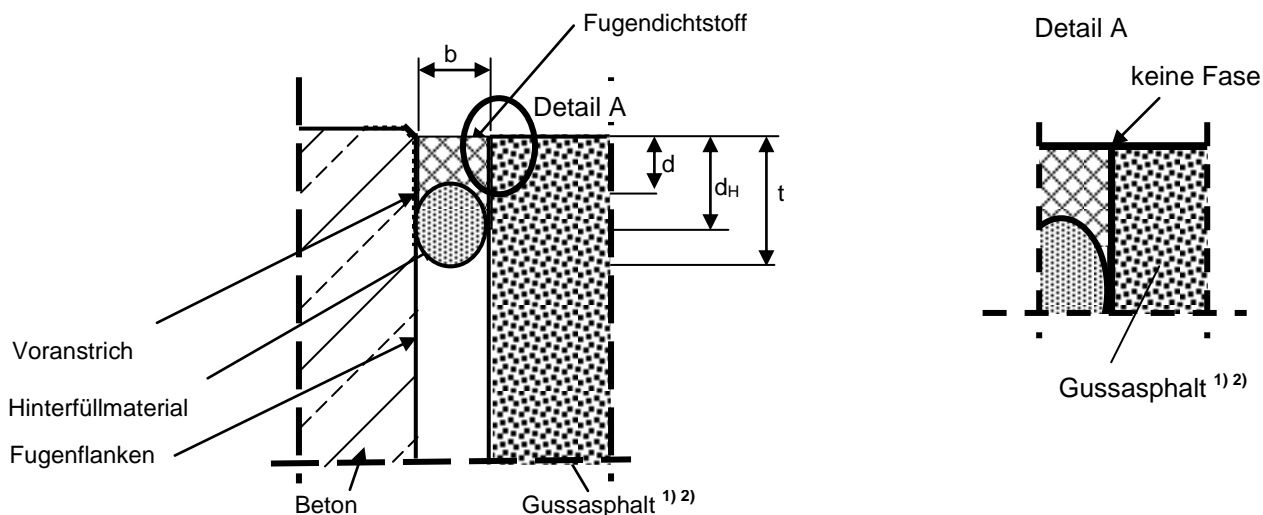
Abbildung 1: befahrbare Fugenausbildung
