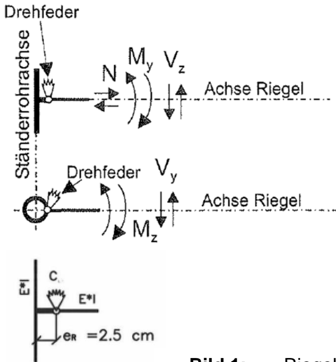
Bild 1: Riegelanschluss
