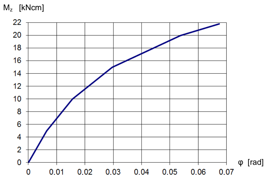
Bild 4: Drehfedersteifigkeit im Rohr-Riegelanschluss bei Biegemoment in der vertikalen Ebene
