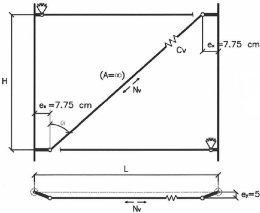
Bild 2: Vertikaldiagonalenanschluss
