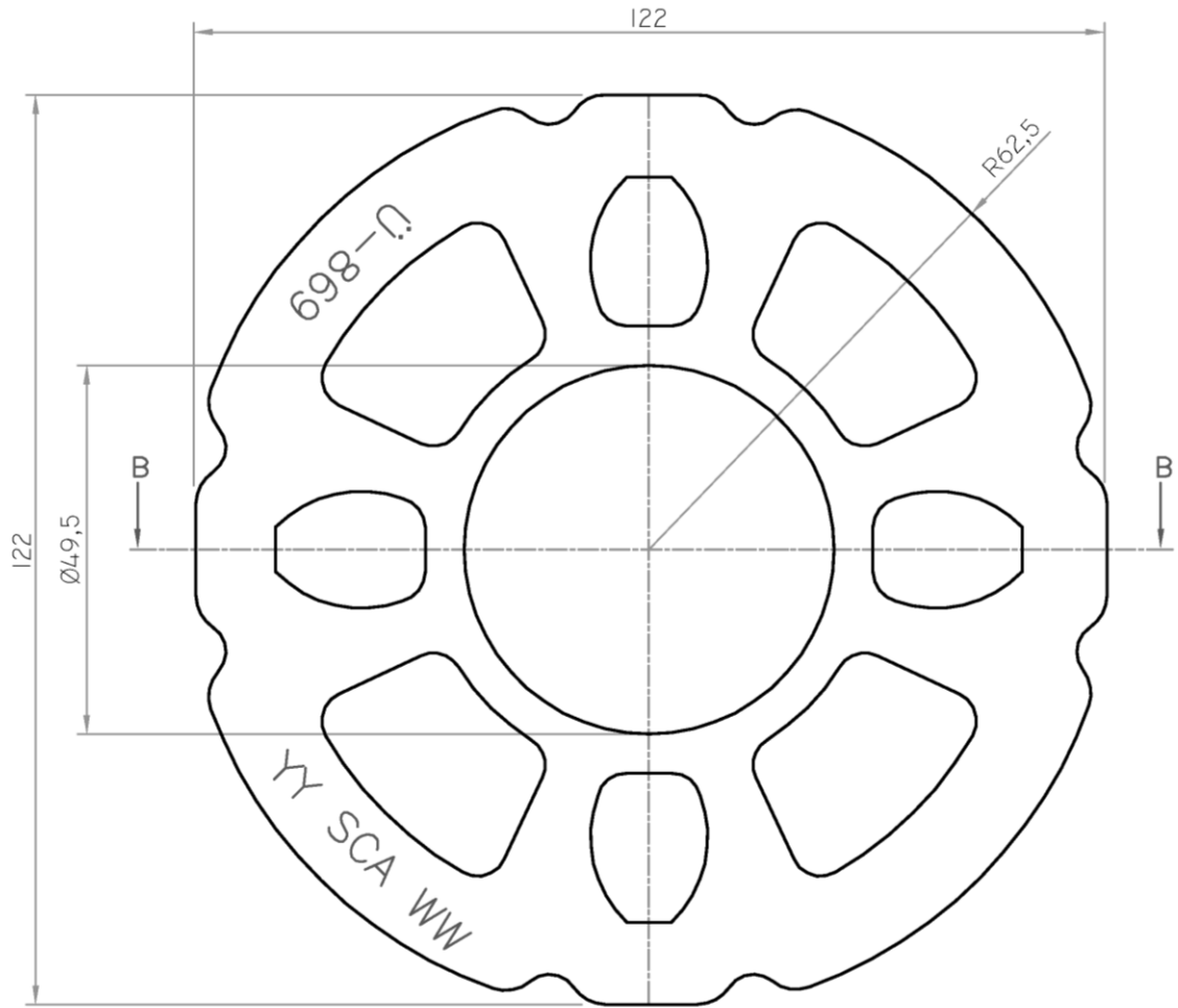
SCHNITT B-B:
