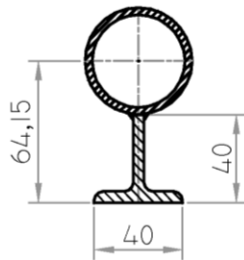
SCHNITT: A-A
