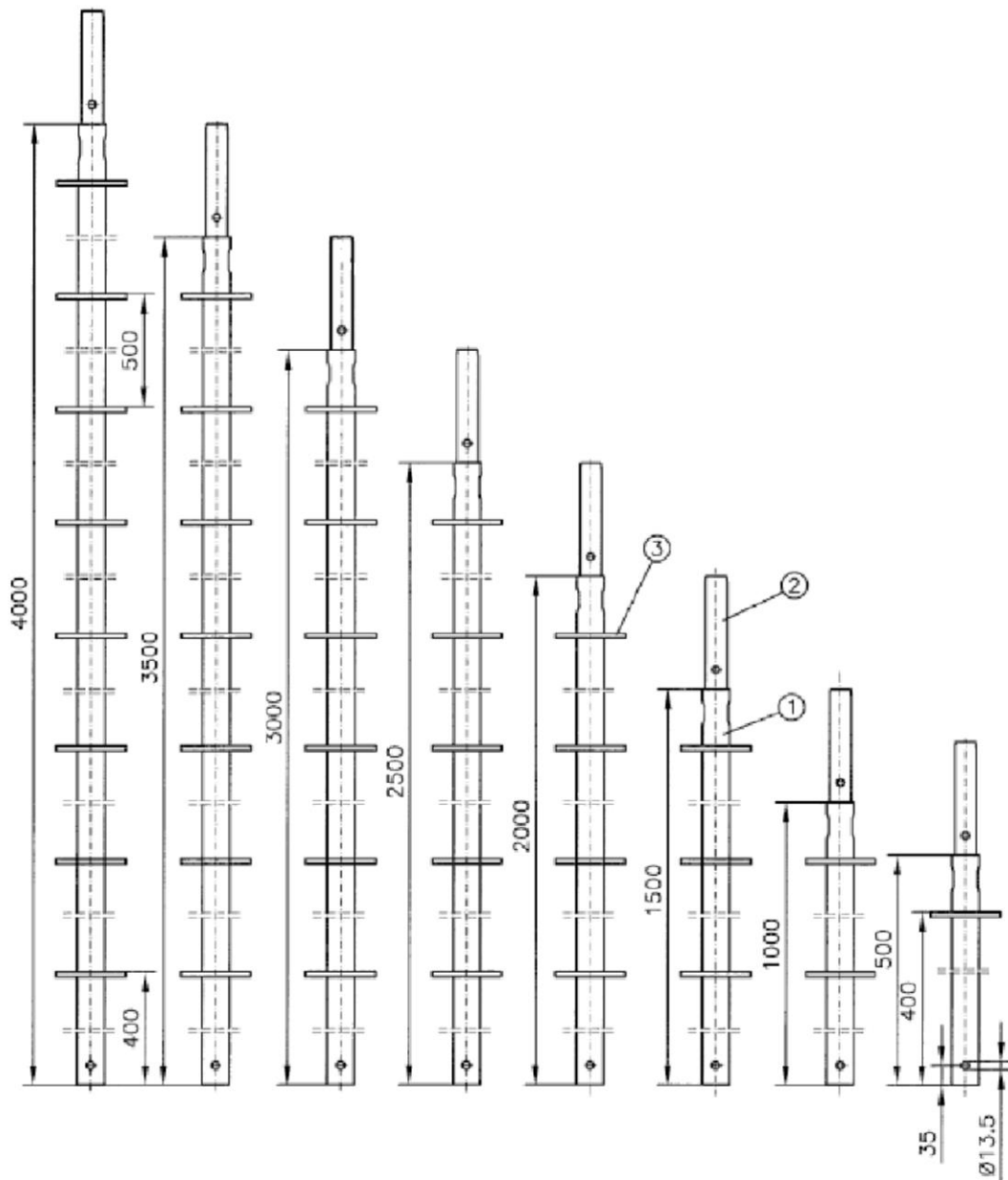
Einpressung der Rohrverbinder und Kennzeichnung siehe Anlage B, Seite 46
