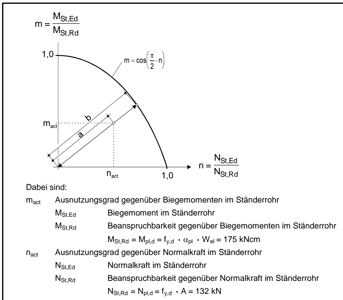
Bild 1: Vektorieller Ausnutzungsgrad im Ständerrohr
