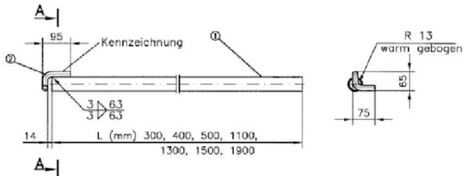
Schnitt A-A
