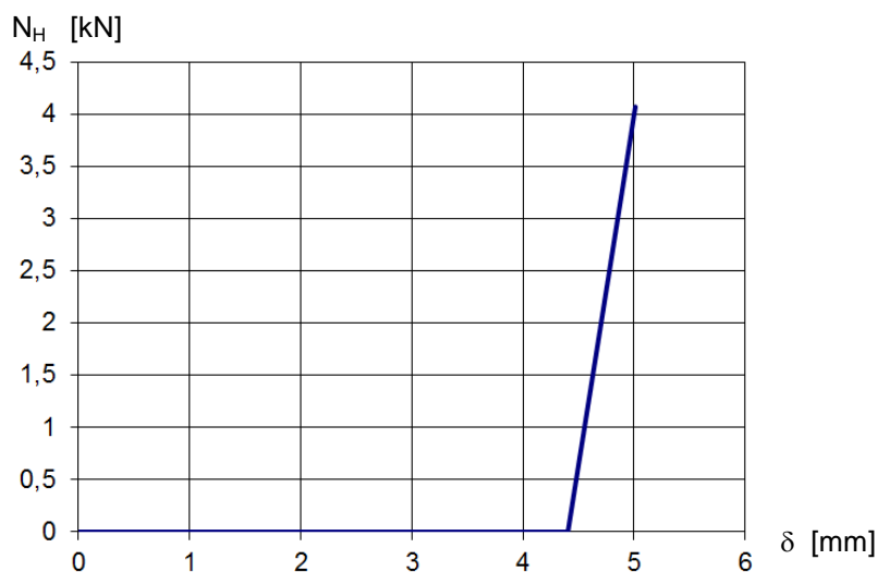
Bild 5: Wegfedersteifigkeit im Anschluss einer Horizontaldiagonalen nach Anlage B, Seiten 8 und 65
