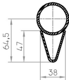
SCHNITT: A-A
