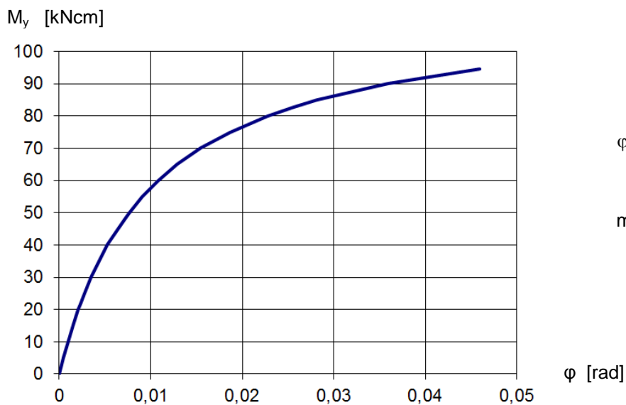
Bild 3: Drehfedersteifigkeit im Rohr-Riegelanschluss bei Biegemoment in der vertikalen Ebene
