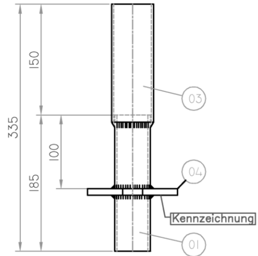
Ausführung Verlängert
