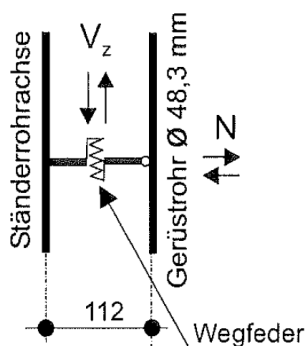
Bild 7: Statisches Modell für die Keilkopfkupplung starr nach Anlage B, Seite 93
