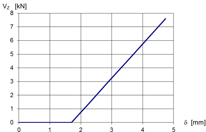
Bild 6: Wegfedersteifigkeit im Anschluss einer Keilkopfkupplung starr nach Anlage B, Seite 93 in der Ständerrohrachse
