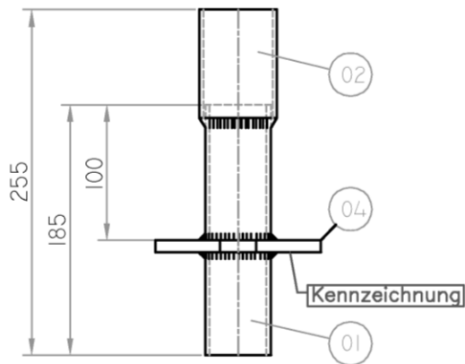
Ausführung Standard
