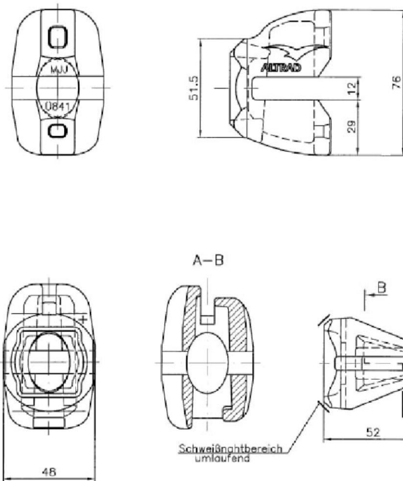
Anschlusskopf für Keilkopfkupplung
