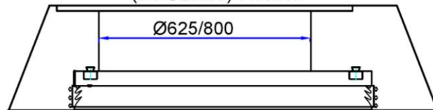
Beton-Konus mit PU-Auskleidung i.A. an DIN4034-1 Einsatzbereich: begehbare und befahrbare (bis SLW60) Flächen
