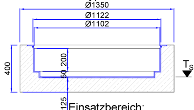
Betonunterteil (C40/50) Typ IV
