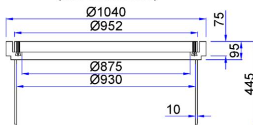
Kunststoffabdeckung aus PO/PE Einsatzbereich: begehbare Fläche (z.B. Grünfläche)
