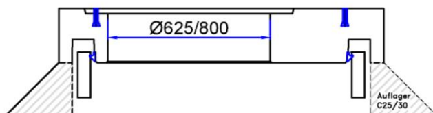
Beton-Abdeckplatte ohne PU-Auskleidung i.A. an DIN4034-1 Einsatzbereich: begehbare und befahrbare (bis SLW60) Flächen
