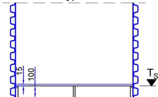
Kunststoffunterteil (PVC-U) Typ III
