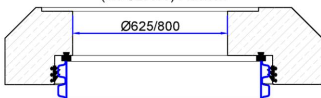
Beton-Abdeckplatte mit PU-Auskleidung i.A. an DIN4034-1 Einsatzbereich: begehbare und befahrbare (bis SLW60) Flächen
