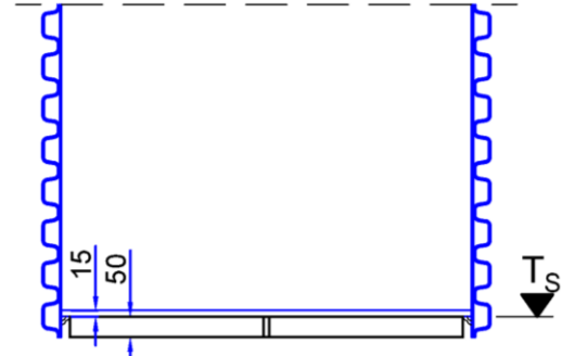
Kunststoffunterteil (PVC-U) Typ II
