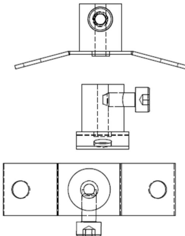
Halterung Temperatursensor
